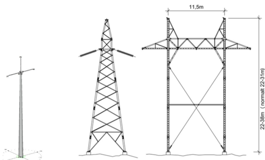
Figur 5: Skisse av enfasemast (venstre) og innvendig bardunert forankringsmast sett fra siden og forfra. Omsøkte maste vil bli henholdsvis ca. 16 m og 25 m høye.
