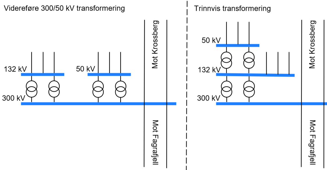
Figur 11: Videreføring av transformering fra 300 til 50 kV gir behov for flere felt på 300(420) kV.
