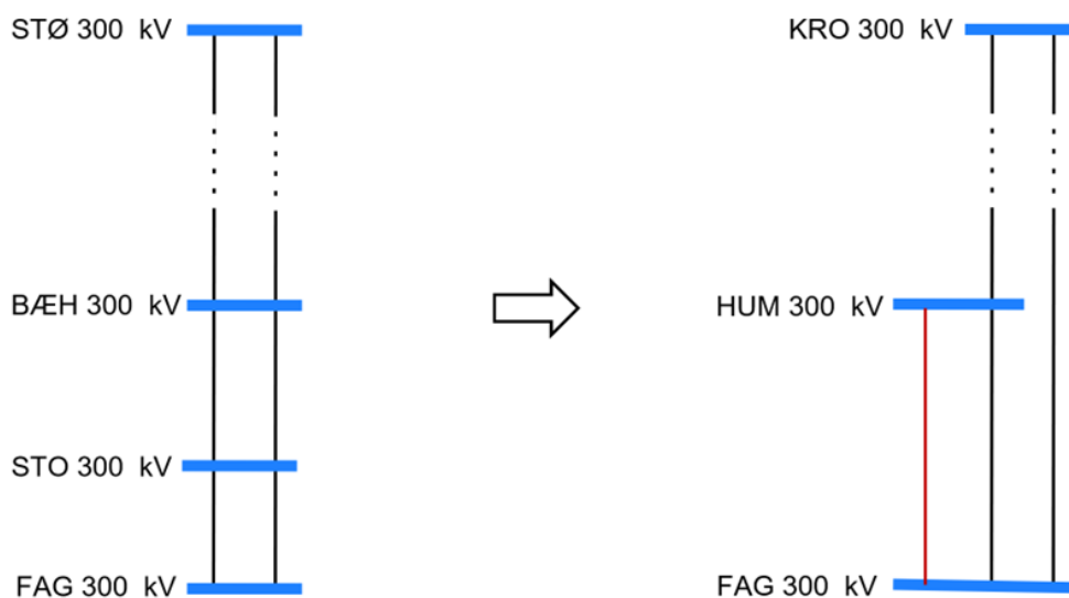
Figur 12: Illustrasjon av dagens situasjon (til venstre) og omsøkt løsning (til høyre) der en ledning mellom Fagrafjell og Krossberg går forbi Humleberget. Rød strek angir ny ledning fra Fagrafjell til Humleberget.
