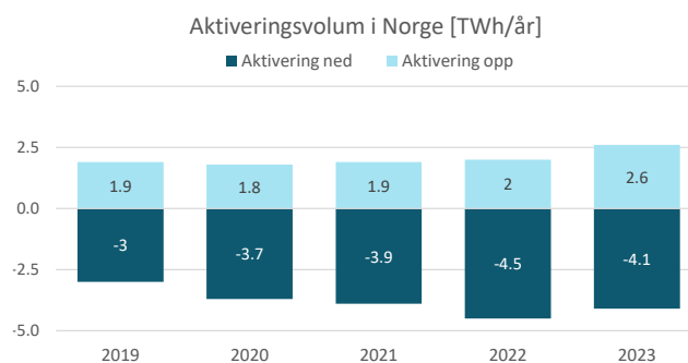
Figur 3 Aktiverte reserver i Norge per år. Fleksibiliteten i norske magasinverk brukes i større andel av tiden til nedregulering
