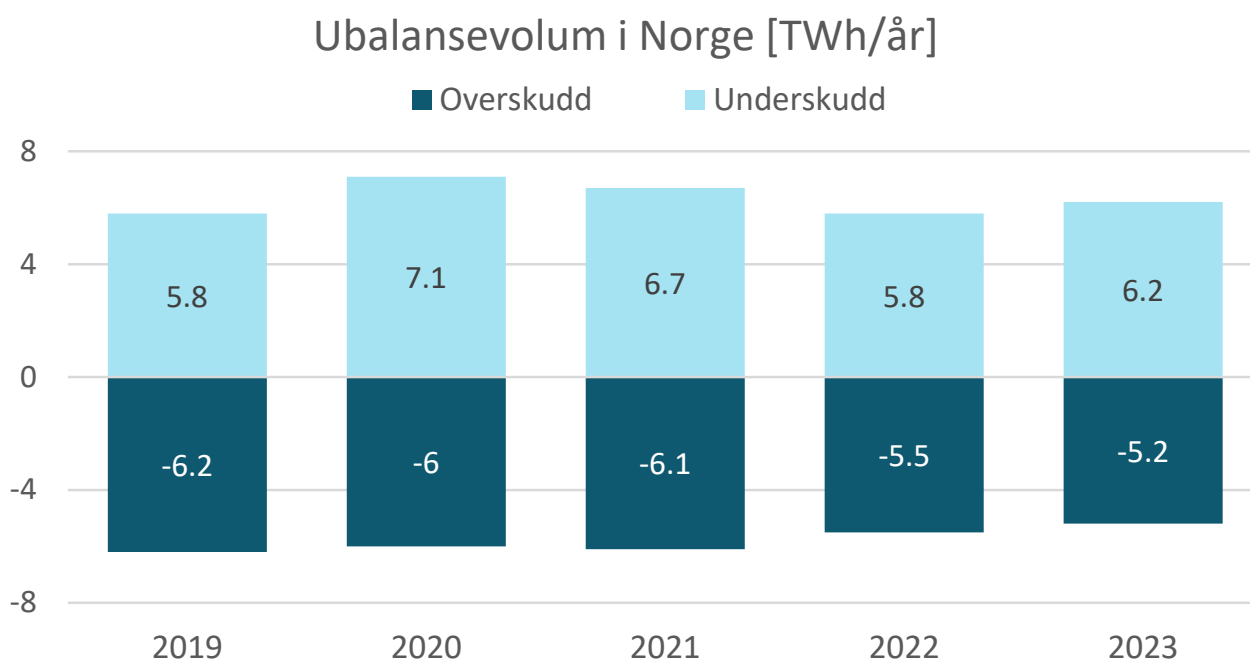
Figur 4 Utvikling i ubalansevolumer hos norske aktører
