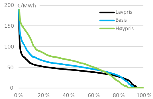
Figur 75: Varighetskurve for priser i NO2 i Basis, Høypris, Lavpris for 2040 i LMA 2024.
