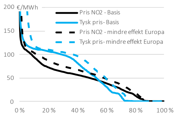
Figur 86: Varighetskurve for prisen i NO2 og Tyskland i Basis og med mindre regulerbar effekti i Europa.
