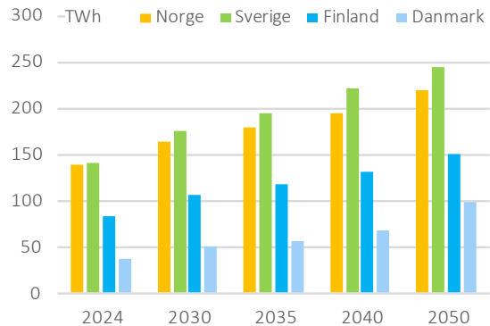
Figur 62: Fordeling av forbruk per land i Medium.
