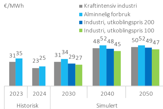
Figur 101: Betalt kraftpris for ulike typer forbruk i NO4. Alle verdier er gjennomsnittspotprisen før fratrukk av strømstøtte.
