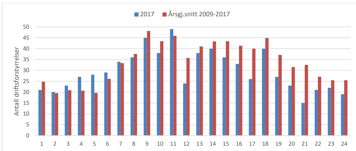
Figur 2.18 Fordeling av driftsforstyrrelser over døgnet
