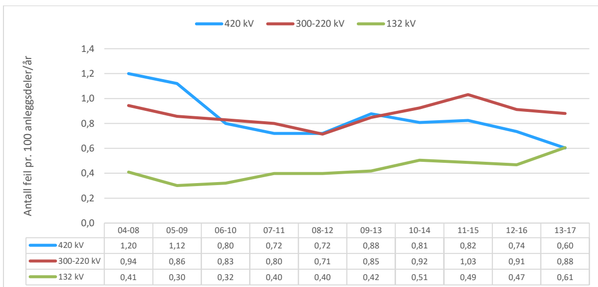
Figur 3.14 Feilfrekvens for effektbryter vist som glidende 5 års gjennomsnitt
