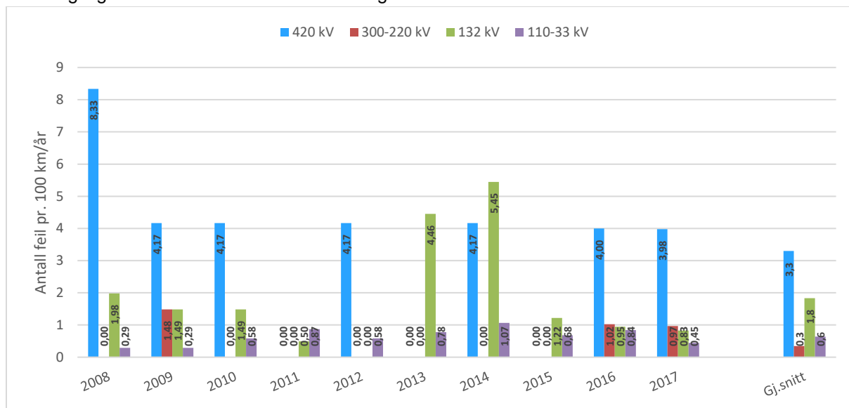
Figur 3.8 Feilfrekvens for kabel fordelt på år og spenningsnivå
