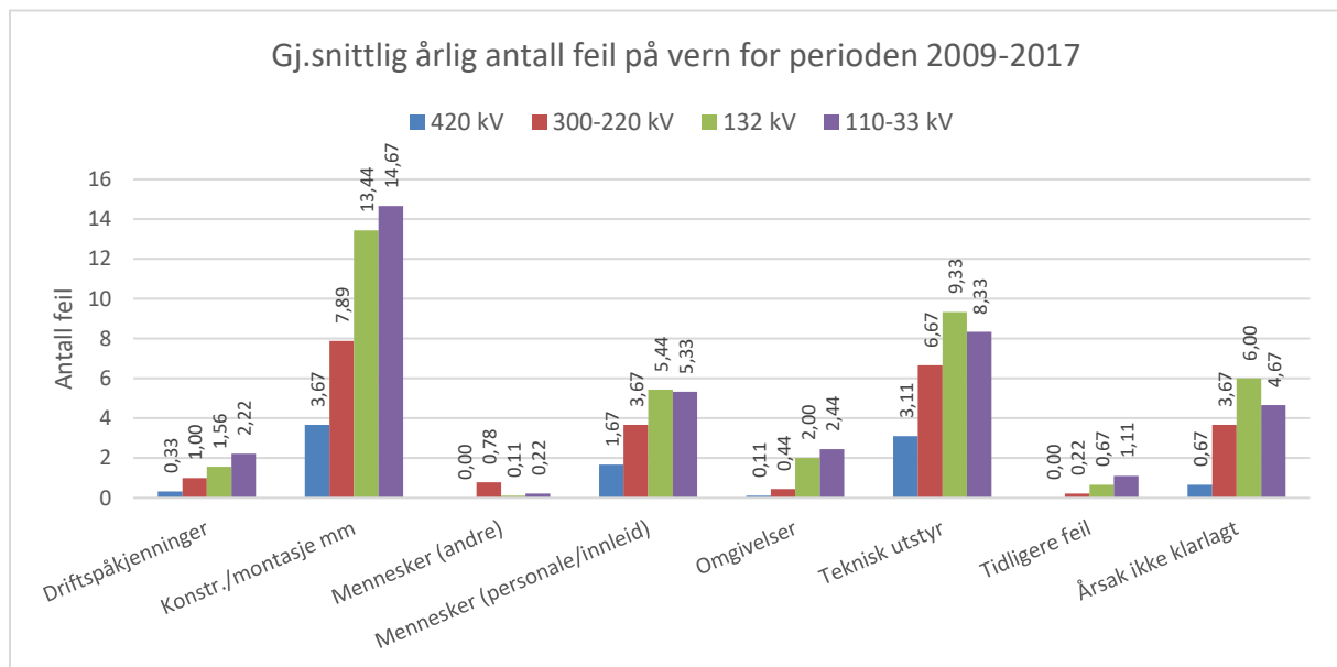
Figur 3.16 Gjennomsnittlig årlig antall feil på vern fordelt på utløsende årsak for perioden 2009-2017
