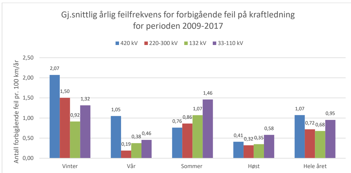
Figur 3.4 Gjennomsnittlig årlig feilfrekvens for forbigående feil på kraftledning fordelt på årstid for perioden 2009-2017
