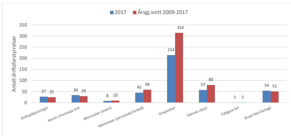
Figur 2.8 Antall driftsforstyrrelser på nettanlegg fordelt på utløsende årsak
