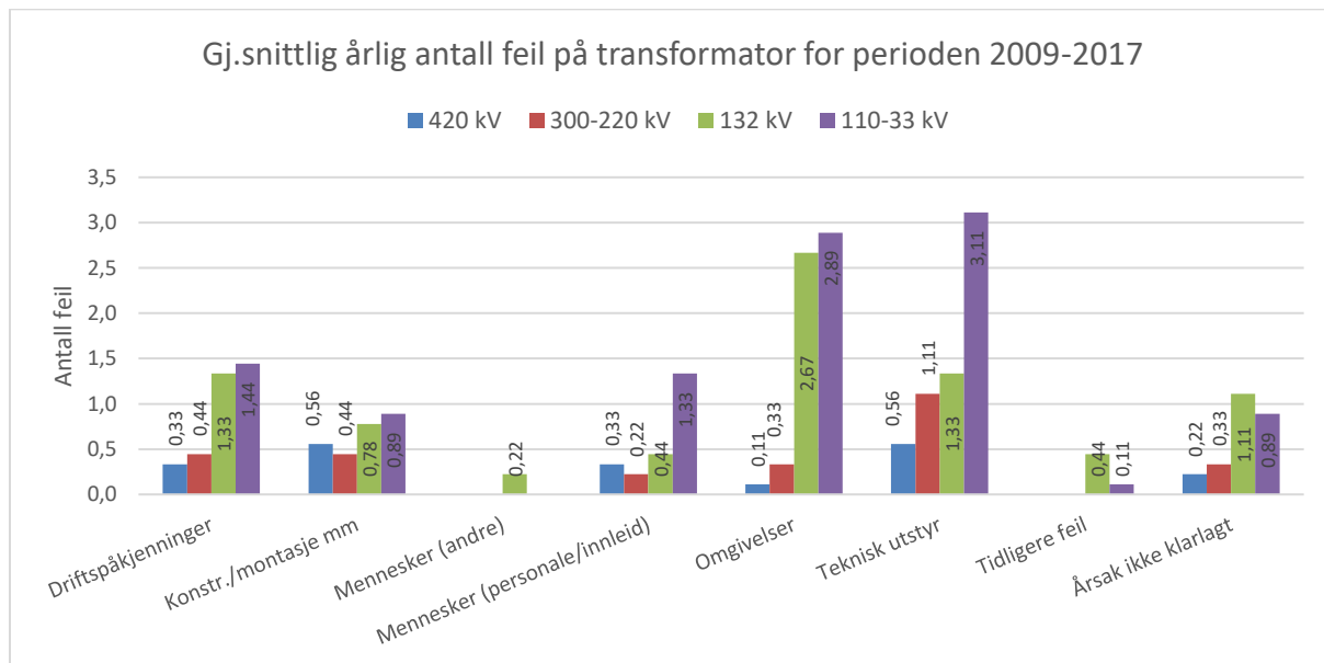
Figur 3.12 Gjennomsnittlig årlig antall feil på krafttransformator fordelt på utløsende årsak for perioden 2009-2017
