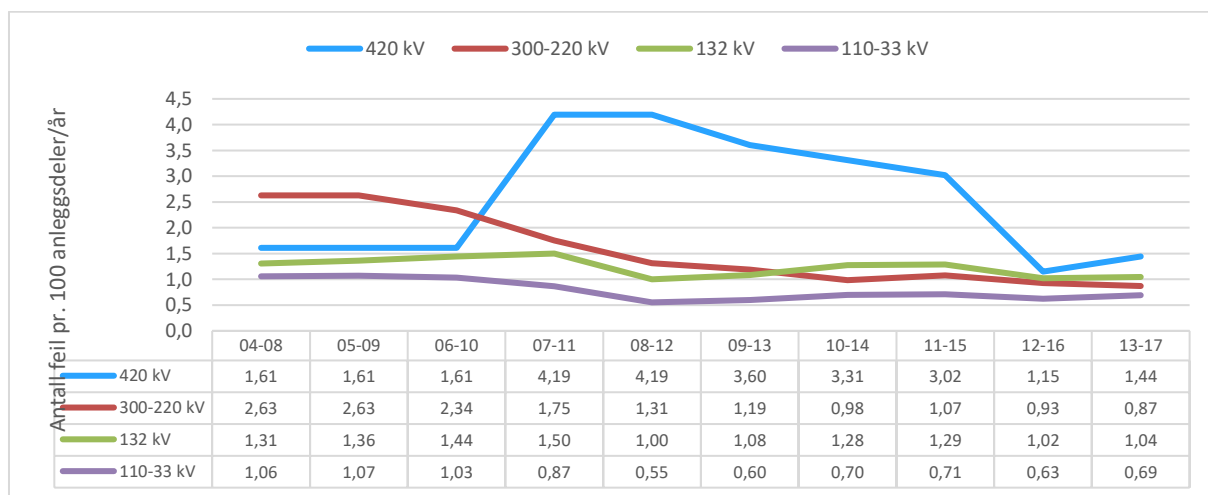
Figur 3.11 Feilfrekvens for krafttransformator vist som glidende 5 års gjennomsnitt
