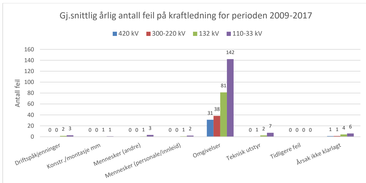
Figur 3.6 Gjennomsnittlig årlig antall feil på kraftledning fordelt på utløsende årsak for perioden 2009-2017
