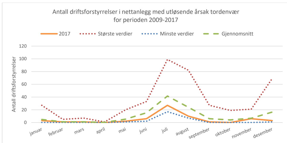
Figur 2.12 Utløsende årsak tordenvær fordelt over året for nettanlegg i perioden 2009-2017
