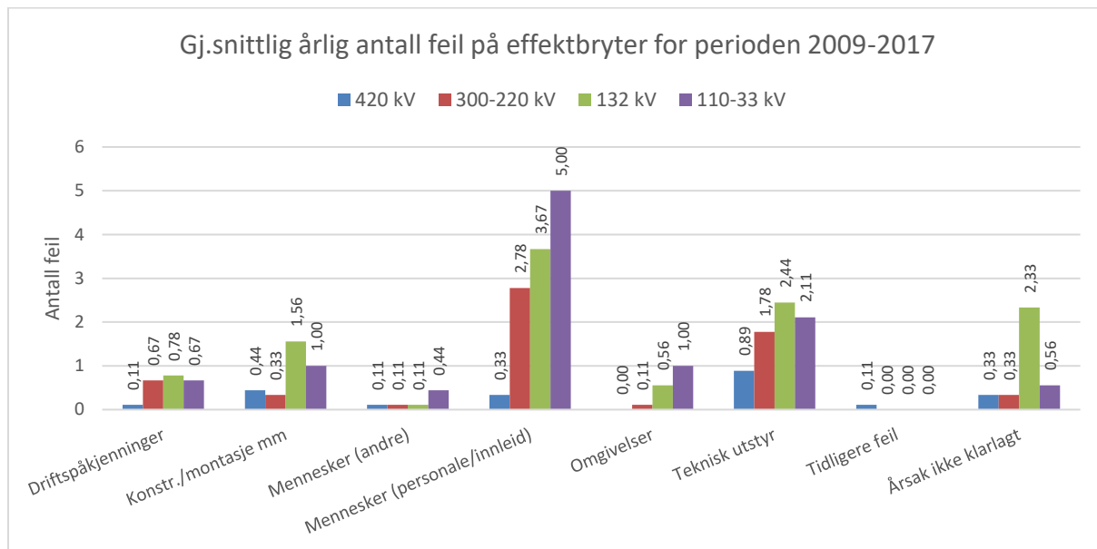
Figur 3.15 Gjennomsnittlig årlig antall feil på effektbryter fordelt på utløsende årsak for perioden 2009-2017
