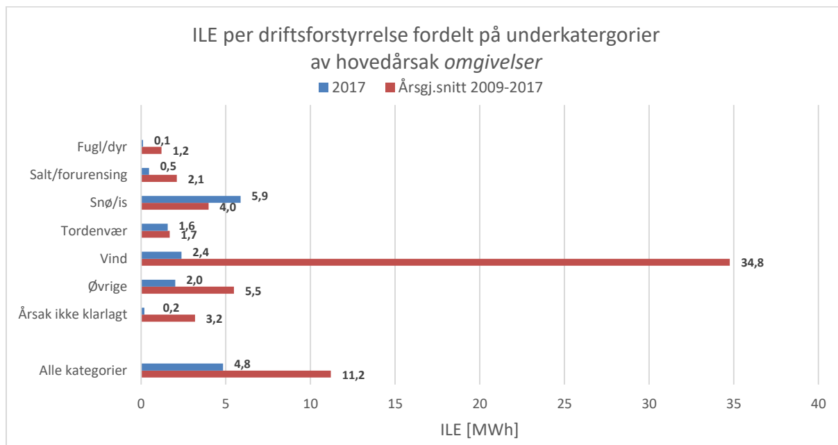
Figur 2.11 Gjennomsnittlig ILE per driftsforstyrrelse fordelt på utløsende årsak innen hovedgruppe omgivelser. (Datagrunnlag er alle driftsforstyrrelser, også de som ikke har medført avbrudd).
