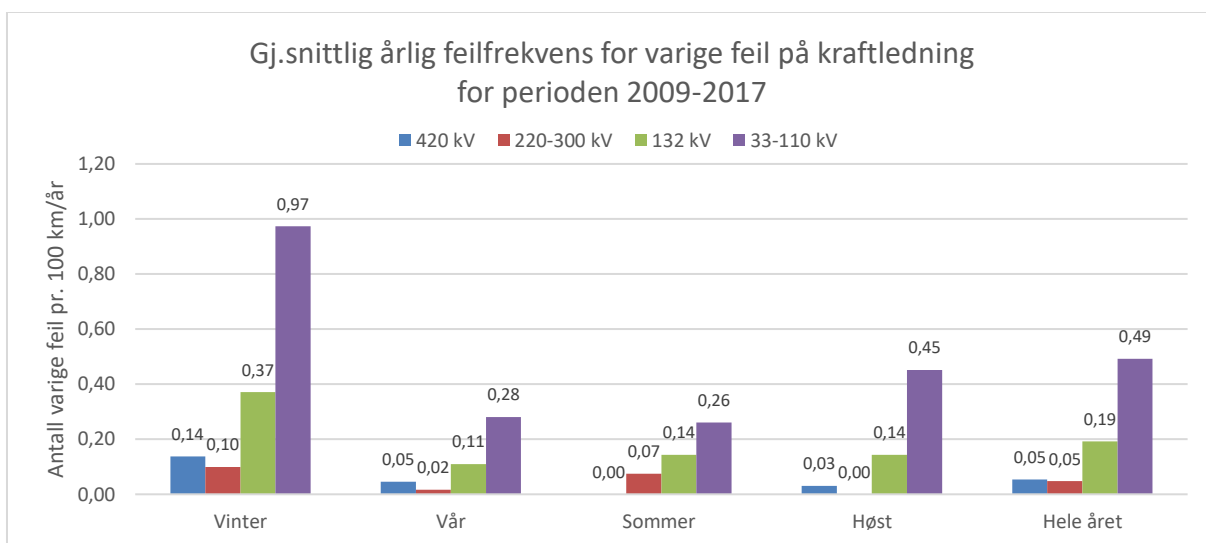
Figur 3.5 Gjennomsnittlig årlig feilfrekvens for varige feil på kraftledning fordelt på årstid for perioden 2009-2017
