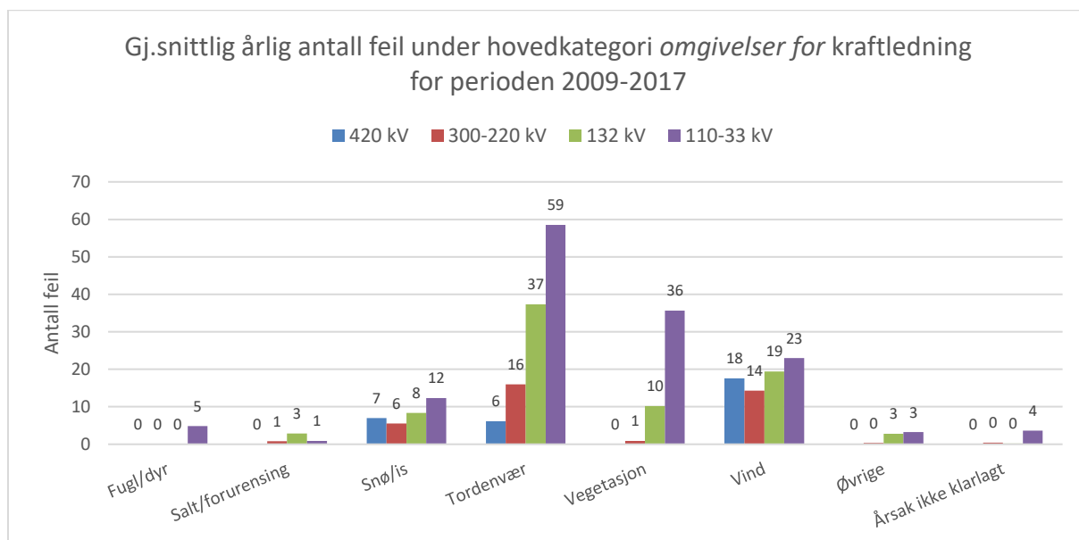
Figur 3.7 Gjennomsnittlig årlig antall feil på kraftledning fordelt på underkategorier av den utløsende årsaken omgivelser for perioden 2009-2017
