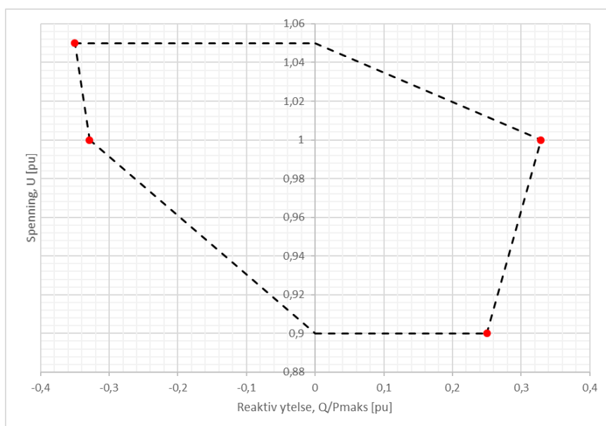
FIGUR 16-3: REAKTIV YTELSE FOR EN KRAFTPARK VED VARIERENDE SPENNING, I U - Q/P_{maks} -PROFIL. RØDE PUNKTER ANGR VERDIENE SOM SKAL DOKUMENTERES.
