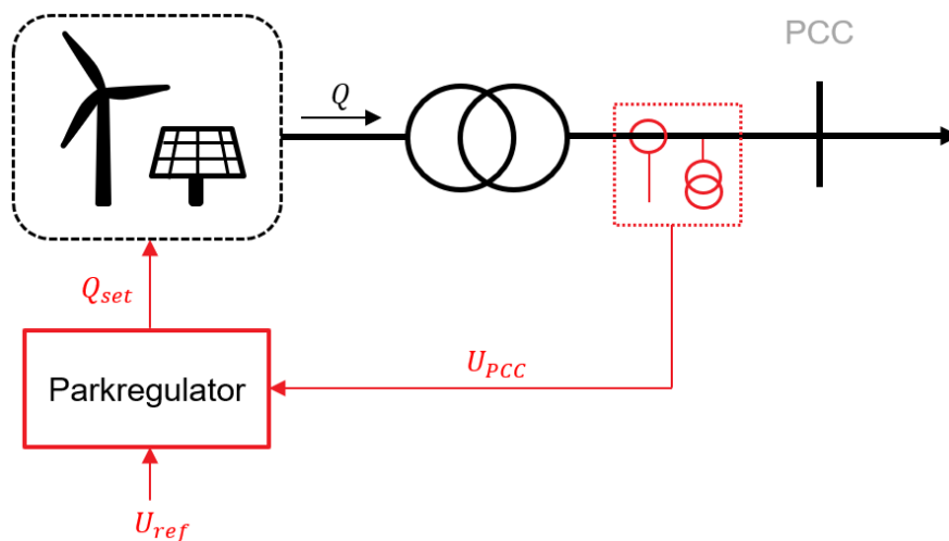
FIGUR 16-10: FORENKLET ILLUSTRASJON AV SPENNINGREGULERING VED TILBAKEKOBLING AV MÅLT NETTSPENNING OG ENDRING I SPENNINGREFERANSE.
