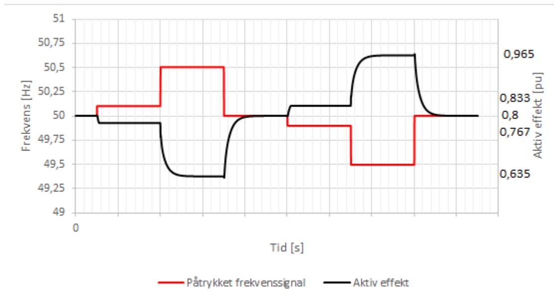
FIGUR 13-42: ILLUSTRASJON AV TEST AV AKTIV EFFEKTTRESPONS (SORT) VED PÅTRYKKE FREKVENSSTEG (RØD).
