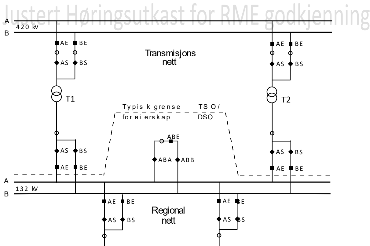
FIGUR 5-2: EKSEMPEL PÅ MINIMUMSLØSNING TIL KOBLINGSANLEGG FOR REGIONALNETTSTASJON TILKNYTTET TRANSMISJONSNETT: LUFTISOLERT ANLEGG MED AB SAMLESKINNE, DOBLE EFFEKTBRYTTERE, SKILLEBRYTTERE OG ENKLE STRØMTRANSFORMATORER, SAMT SAMMENKOBLEBRYTTERE.
