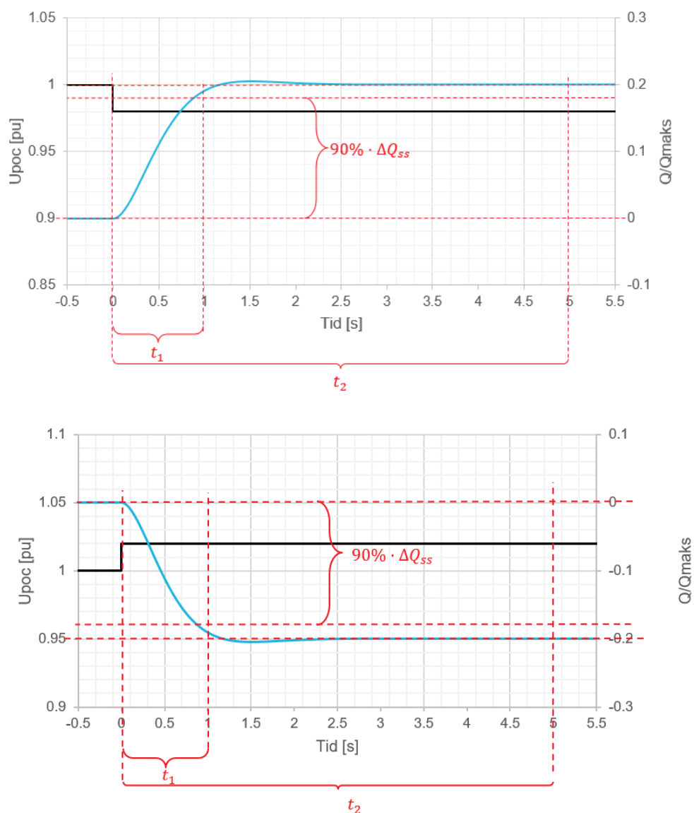
FIGUR 14-6: REAKTIV EFFEKTRESPONS VED STEGVIS ENDRING I SPENNING PÅ HHV -/+ 2\% . KRAV ER MARKERT I RØDSTIPLEDE LINJER.
