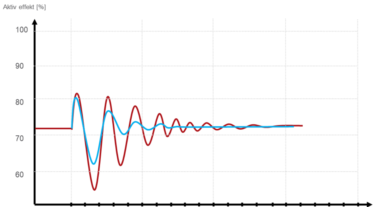
FIGUR 13-51: ILLUSTRASJON AV DEMPETILSATSENS EFFEKT PÅ EFFEKTPENDLINGER ETTER EN PÅTRYKKE SPENNINGSPULS. BLÅ VISER AKTIV EFFEKTRESPONS MED AKTIV DEMPETILSAT, OG RØD VISER AKTIV EFFEKTRESPONS UTEN DEMPETILSAT.
