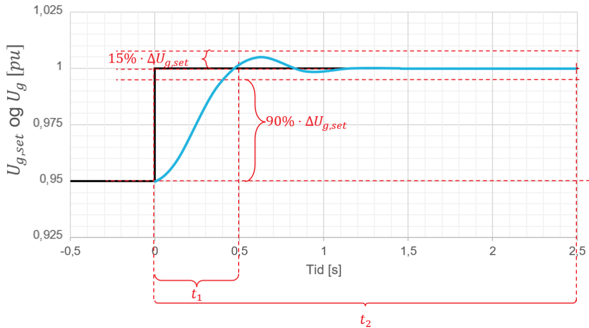
FIGUR 12-8: ILLUSTRASJON AV KRAV TIL UTREGULERINGSTID AV SPENNINGSETPUNKT REFERANSESTEG I POSITIV RETNING FOR MAGNETISERINGSUTSTYR I LUKKET SLØYFE MED ÅPEN EFFEKTBRUYTER FOR SYNKRONE PRODUKSJONSENHETER.
