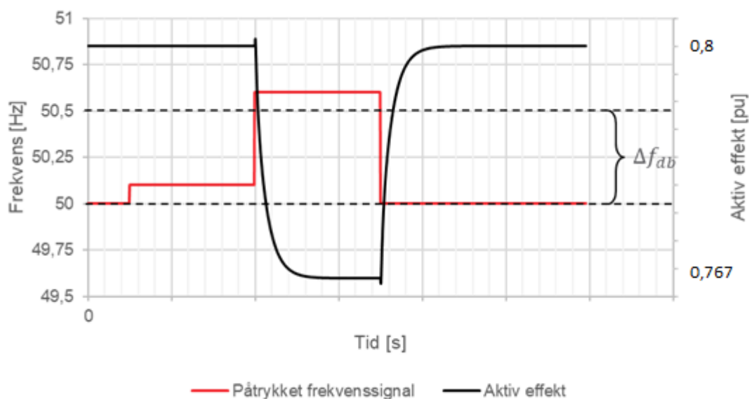
FIGUR 13-43: ILLUSTRASJON AV PRØVE FOR AKTIV EFFEKTPRESPONS (SORT) VED PÅTRYKKET FREKVENSTEG (RØD) MED AKTIVE DØDBÅND (SORT STIPLET LINJE).
