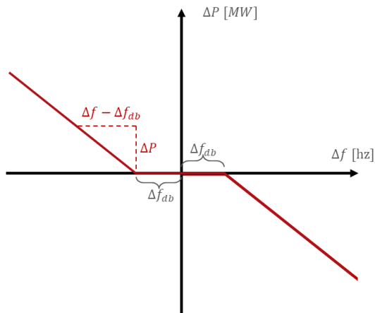
FIGUR 18-2: REGULATORRESPONS SOM FUNKSJON AV FREKVENSI I FREKVENSRULERINGSMODUS FOR HVDC-SYSTEMER
