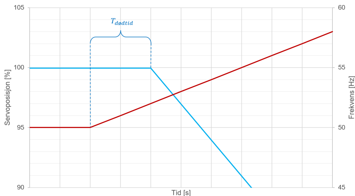
FIGUR 13-24: ILLUSTRASJON AV PRØVE FOR DOKUMENTASJON AV DØDTID I SERVOSYSTEM VED FULLASTAVSLAG.
