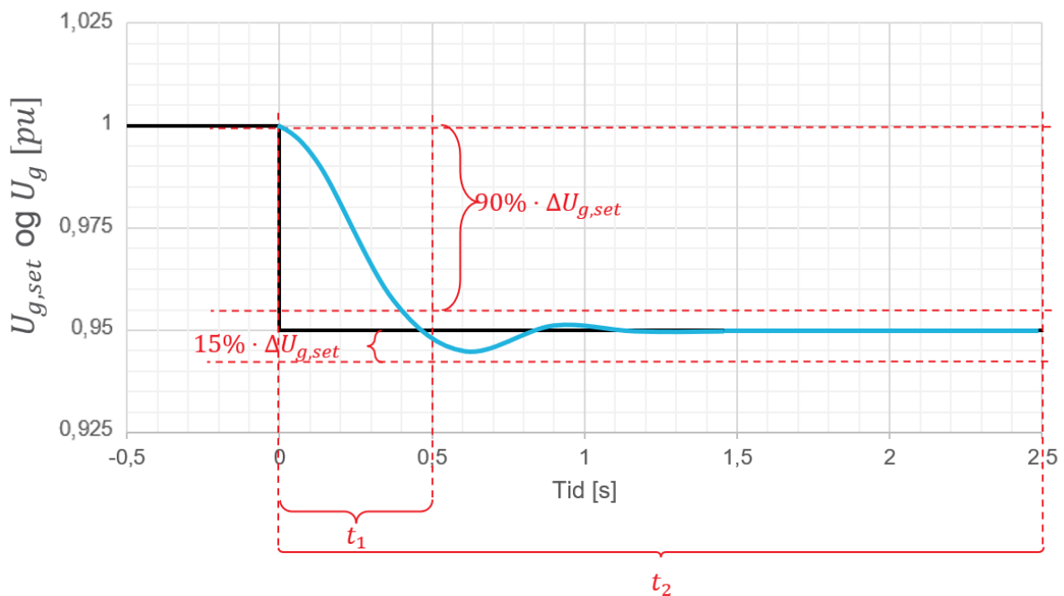
FIGUR 12-9: ILLUSTRASJON AV KRAV TIL UTREGULERINGSTID VED SPRANG AV SPENNINGSETPUNKTREFERANSESTEG I NEGATIV RETNING FOR MAGNETISERINGSUTSTYR I LUKKET SLØYFE MED ÅPEN EFFEKTBRUYTER FOR SYNKRONE PRODUKSJONSENHETER.
