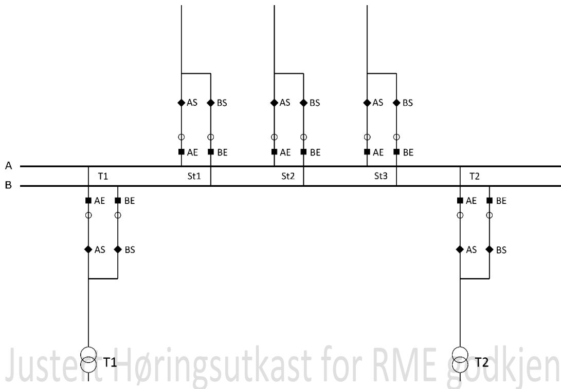
FIGUR 5-1: EKSEMPEL PÅ STASJONSLØSNING MED HØYESTE FLEKSIBILITET I TRANSMISJONSNETT FOR LUFTISOLERT ANLEGG BASERT PÅ TO BRYTERE OG TO STRØMTRANSFORMATORER MED AB SKINNE.
