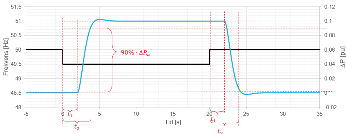
FIGUR 14-5: KRAV TIL FREKVENSTEGRESPONS FOR KRAFTPARKER, HER VED 10 % STATIKK OG FREKVENSTEG PÅ 0,5 Hz.
