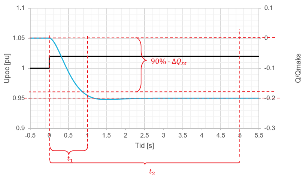
FIGUR 16-22: ILLUSTRASJON AV PRØVER FOR DOKUMENTASJON AV KRAV TIL UTREGULERINGSTID AV SPENNINGREFERANSESTEG I NEGATIV RETNING FOR KRAFTPARKER.
