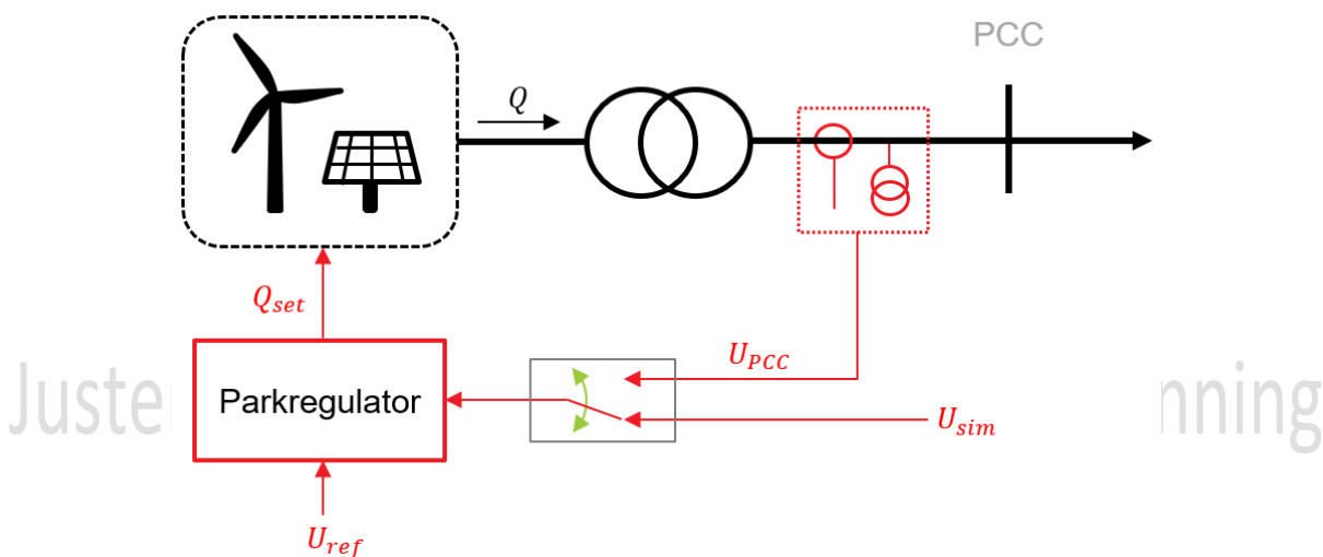
FIGUR 16-13: FORENKLET ILLUSTRASJON AV SPENNINGREGULERING VED EKSTERNT SIMULERT SIGNAL FOR NETTSPENNING UTEN TILBAKEKOBING AV MÅLT NETTSPENNING.
