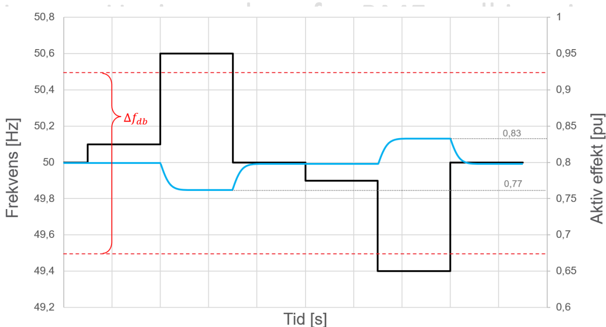
FIGUR 13-26: TEST AV EFFEKTRESPONS (BLÅ) VED PÅTRYKKET FREKVENSSPRANG (SORT) MED AKTIVT DØDBÅND (STIPLT LINJE).
