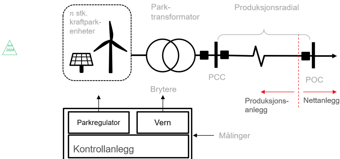
FIGUR 14-1: ILLUSTRASJON AV HOVEDKOMPONENTER I EN KRAFTPARK, HER VED EN VINDPARK ELLER SOLPARK, MED NOTASJONER. RØD STIPLET LINJE INDIKERER SKILLET MELLOM HVOR DET STILLES KRAV I DEL II NETTANLEGG OG DEL IV PRODUKSJONSENHETER.
