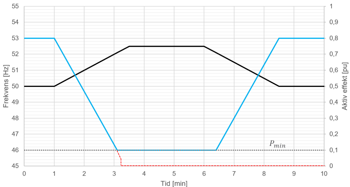
FIGUR 16-9: AKTIV EFFEKTRESPONS (BLÅ) VED PÅTRYKKET FREKVENSRAMPE (SORT). VED 52,5 Hz HOLDER PARKEN SETTPUNKTET P_{min} ISTEDEFOR Å KOBLE UT ELLER GÅ TIL STOPP (RØD STIPILET LINJE).
