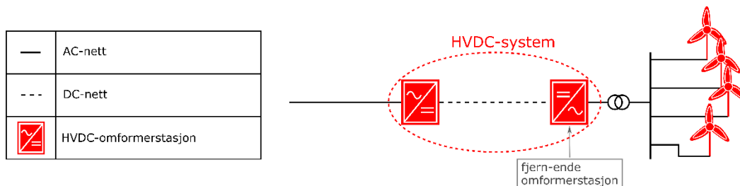
FIGUR 17-2: ILLUSTRASJON AV HVDC-SYSTEM MED FJERN-ENDE HVDC-OMFORMER
