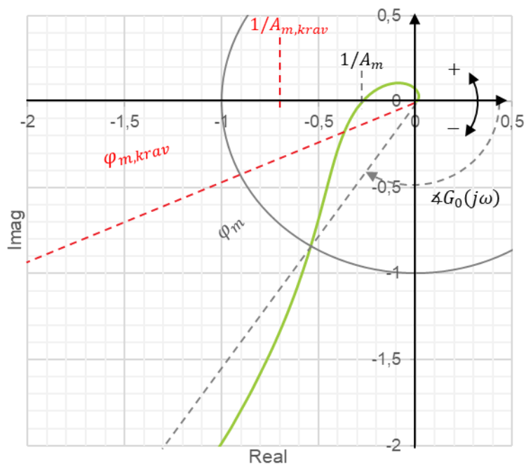
FIGUR 13-8: ILLUSTRASJON AV FREKVENSPANSRESPONSEN (GRØNN) TIL G_o(s) , REF. LIGNING 13-1, I ET NYQUIST-DIAGRAM, HVILKET UTTRYKKER STABILITETEN TIL SYSTEMET. RØDSTIPLEDE LINJER INDIKERER KRAVENE TIL STABILITETSMARGIN. GRÅSTIPLEDE ER FAKTISK STABILITETSMARGIN.
