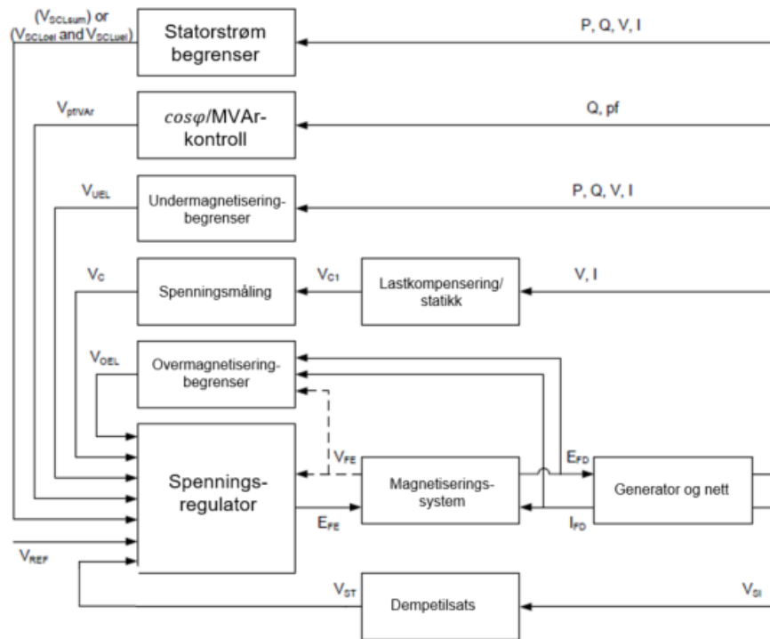
FIGUR 13-14: PRINSIPIELL VIRKEMÅTE TIL SPENNINGREGULATOREN FOR EN SYNKRON PRODUKSJONSENHET [11]. NB; MERK AT BLOKDDIAGRAMMET KUN VISER SPENNINGINNANG TIL DEMPETILSATS. DEMPETILSATS SKAL OGSÅ BENYTTE TURTALL IHT. KRAV I KAPITTEL 12.5.6.
