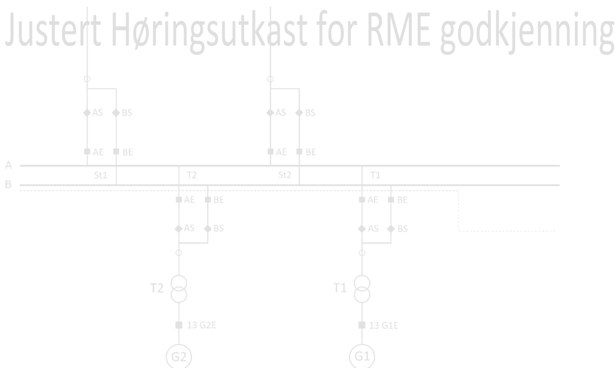
Figur 5-2: Eksempel på stasjonsløsning med høy fleksibilitet for luftisoleret anlegg; AB-samleskinne, doble effektbrytere og enkle strømtransformatorer. Figureksempel slettes i NVF2024.
