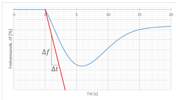
FIGUR 12-3: ILLUSTRASJON AV KRAV TIL FREKVENSDRINGSFASTIGHET. DERSOM FREKVENSLØPET ER OVER DEN RØDE LINJEN, SOM FALLER MED EN FREKVENSDRINGSFASTIGHET \frac{\Delta f}{\Delta t} = 1,5 \text{ Hz/s} , SKAL PRODUKSJONSENHETEN OPERERE NORMALT.
