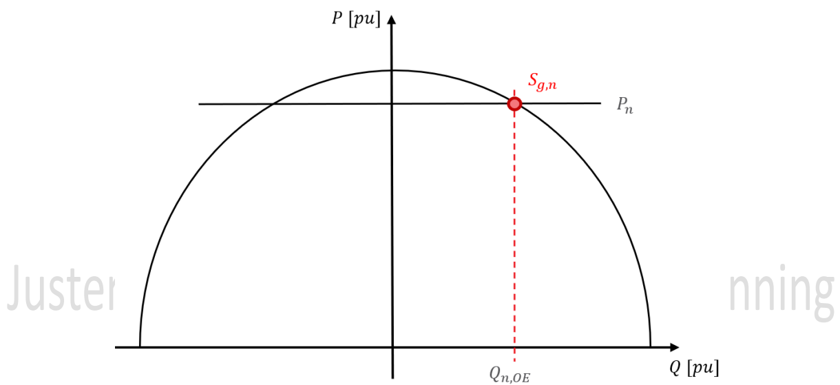
FIGUR 13-32: ILLUSTRASJON AV GENERATORENS DRIFTSPUNKT VED GJENNOMFØRING AV VARMEPRØVE.
