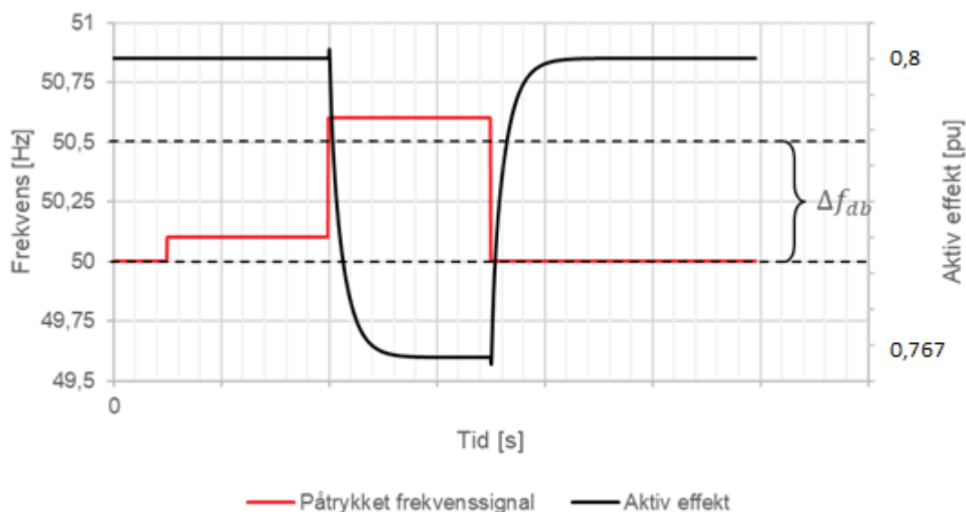
FIGUR 13-25: ILLUSTRASJON AV PRØVE FOR AKTIV EFFEKTRRESPONS (SORT) VED PÅTRYKKET FREKVENNSTEG(RØD) MED AKTIVE DØDBÅND (SORT STIPILET LINJE).
