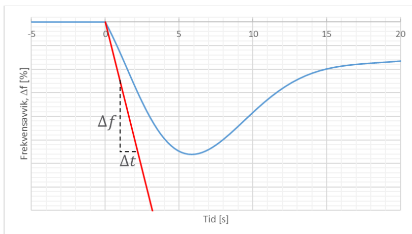
FIGUR 14-2: ILLUSTRASJON AV KRAV TIL FREKVENSENDRINGSHASTIGHET. DERSOM FREKVENSFORLØPET ER OVER DEN RØDE LINJEN, SOM FALLER MED EN FREKVENSENDRINGSHASTIGHET PÅ \frac{\Delta f}{\Delta t} = 1,5 Hz/s , SKAL PRODUKSJONSENHETEN OPERERE NORMALT.
