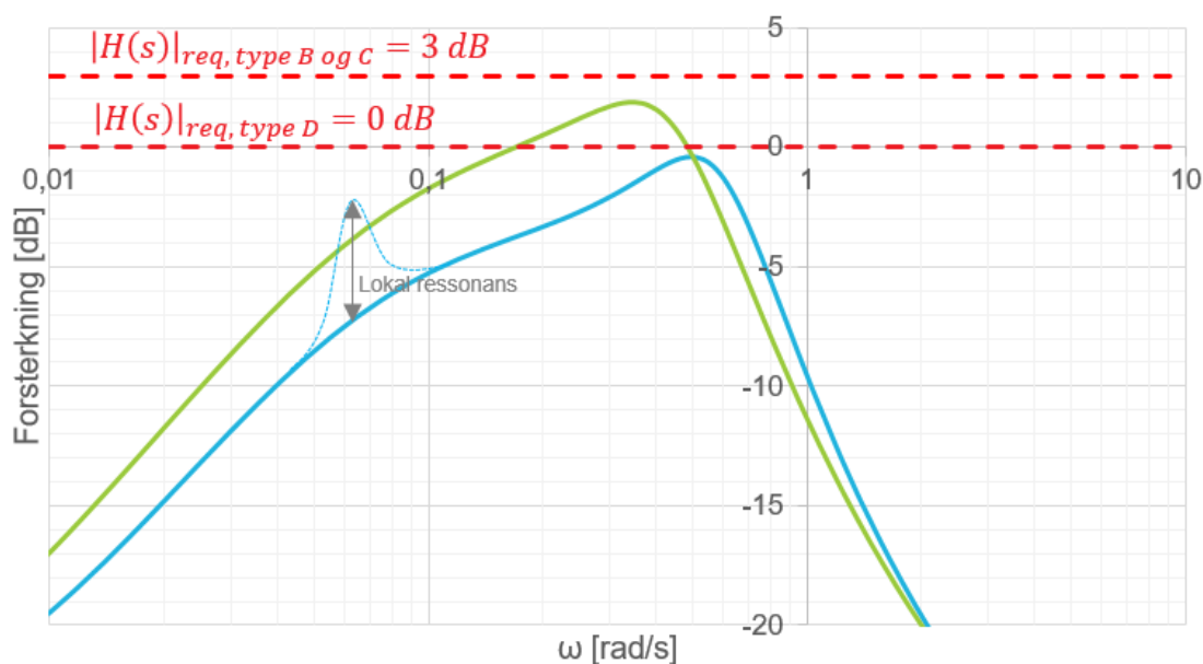
FIGUR 13-11: FREKVENSRRESPONS ILLUSTRERT I FREKVENSPLANET VED 1 % LASTPÅSLAG REFERERT P_{maks} , VED P_{sett} = 0,85 \cdot P_{maks} OG 2 % STATISK. DE RØDE STIPLEDE LINJENE REPRERENTERER KRAVENE TIL MAKSIMALT TRANSIENT FREKVENSAVVIK. GRØNN (TYPE B OG C) OG BLÅ KURVER (TYPE D) ER EKSEMPLER PÅ FREKVENSFORLØP ETTER ET LASTSPRANG PÅ EGET OHMSK NETT.
