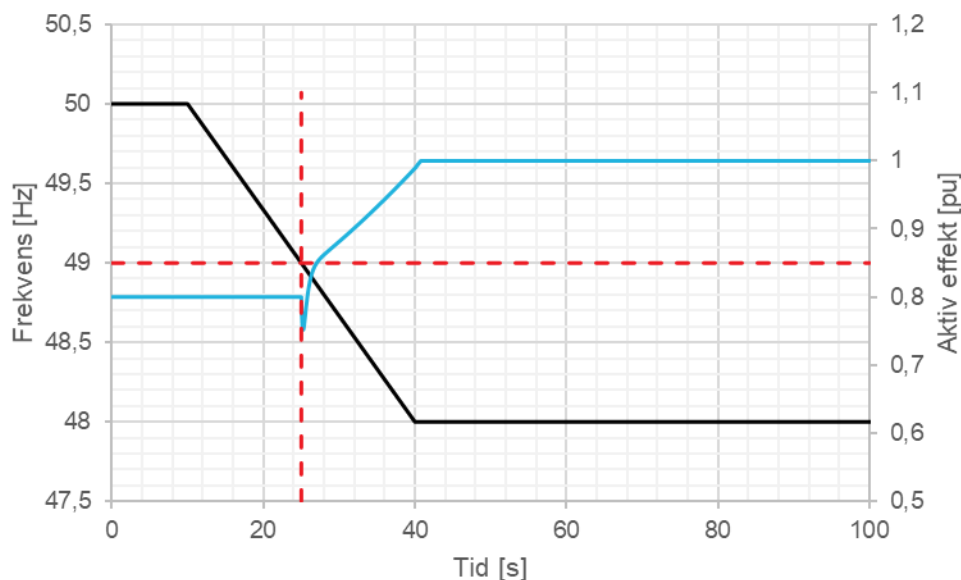
FIGUR 13-27: ILLUSTRASJON AV PRØVE AV AKTIV EFFEKTPRESPONS (BLÅ) VED DETEKSJON AV SEPARATDRIFT VED FREKVENSTERSKEL VED PÅTRYKKET FREKVENSRAMPE (SORT). BLÅ KURVE VISER ENDRING I PARAMETERSETT VED FREKVENNS < 49 Hz.
