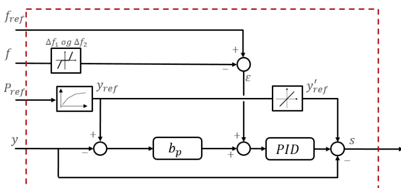
FIGUR 13-6: PRINSIPELL OPPBYGNING AV FREKVENSRGULERING VED TILBAKEFØRING AV SERVOPOSISJON.
