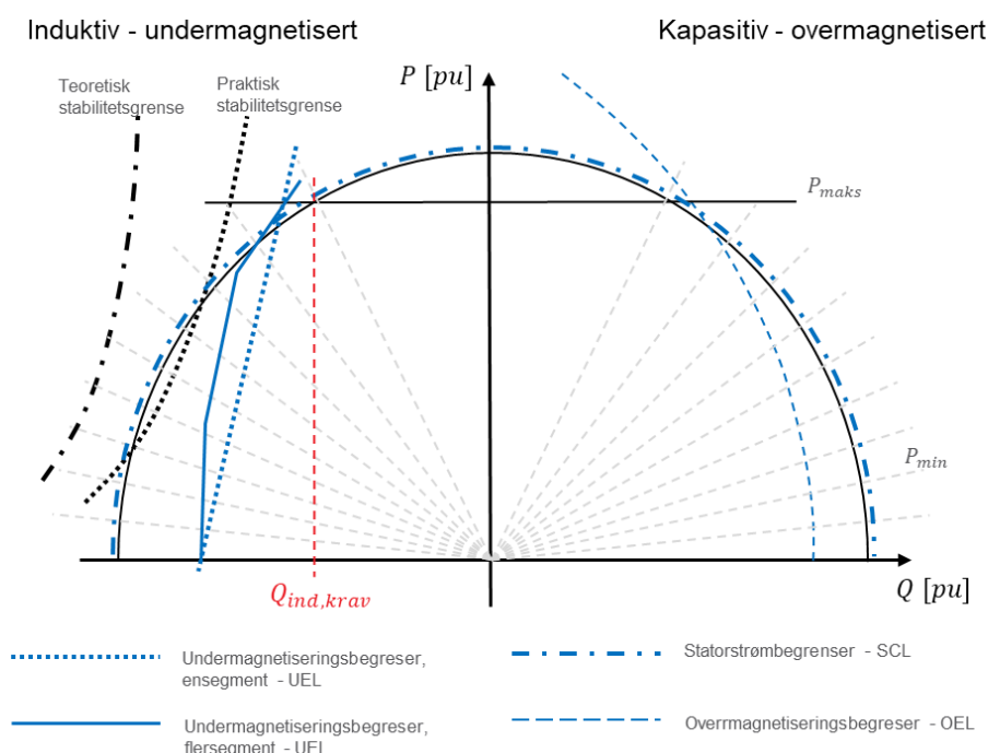
FIGUR 12-10: ILLUSTRASJON AV PRINSIPPER FOR HVORDAN MAGNETISERINGSUTSTYRETS BEGRENERE SKAL INNSTILLES.
