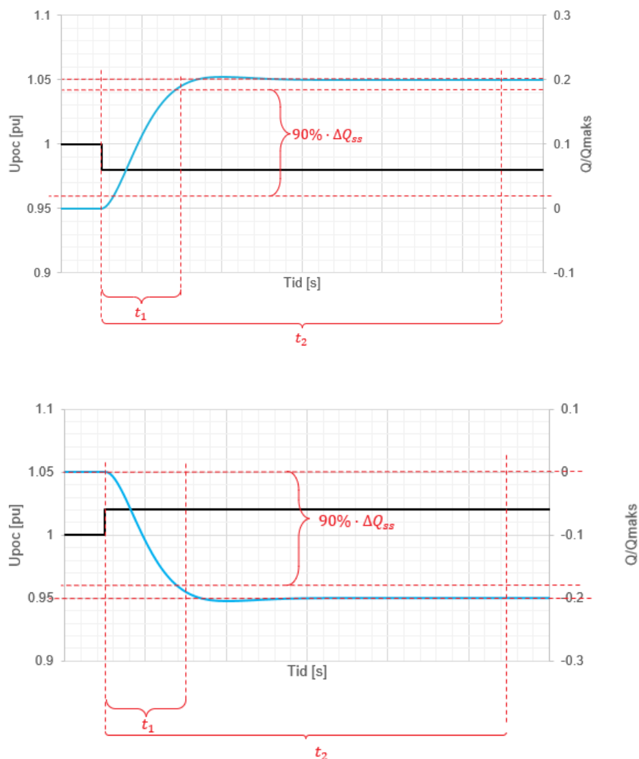
FIGUR 18-6: REAKTIV EFFEKTRSPONS VED STEGVIS ENDRING I SPENNING PÅ HHV -/+ 2\% . KRAV ER MARKERT I RØDSTIPELE LINJER
