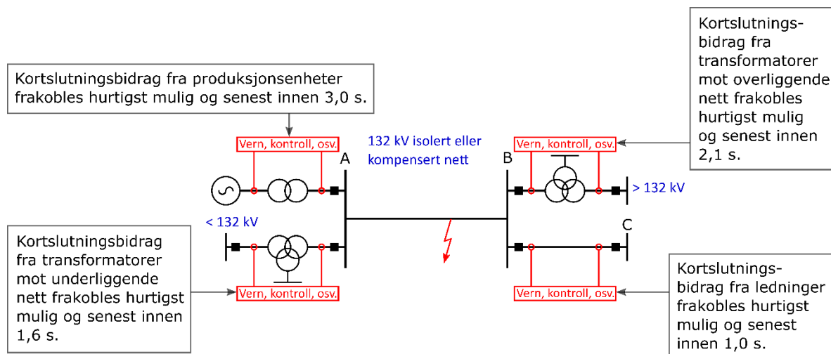
FIGUR 7-3: FRAKOBLING AV FEIL VED VERNSYSTEM- ELLER EFFEKTBYTERSVIKT
