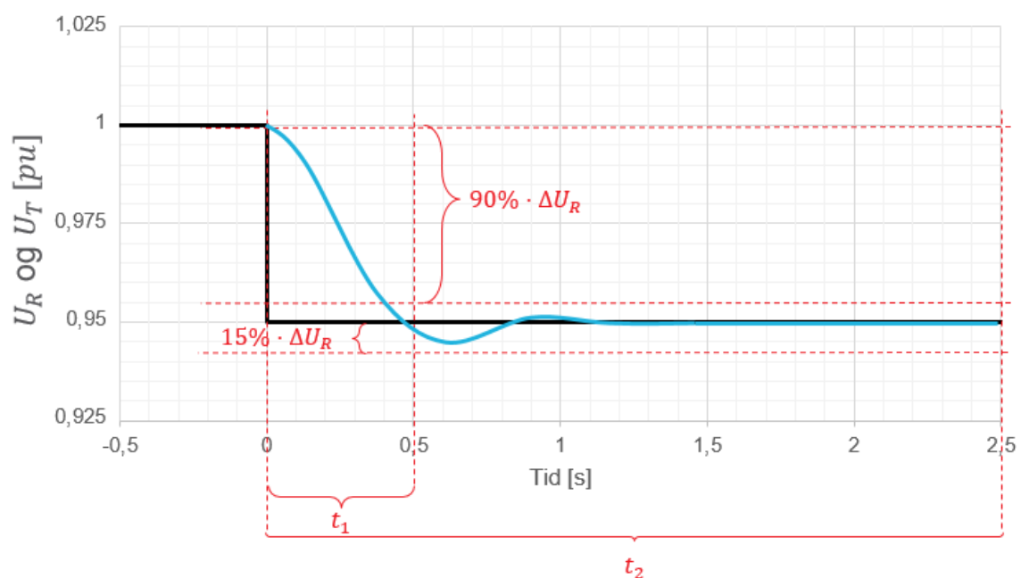
FIGUR 13-16: ILLUSTRASJON AV KRAV TIL UTREGULERINGSTID AV SPENNINGREFERANSESTEG I NEGATIV RETNING FOR MAGNETISERINGSUTSTYR I LUKKET SLØYFE MED ÅPEN EFFEKTBRUYTER FOR SYNKRONE PRODUKSJONSENHETER.
