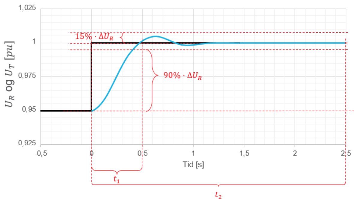
FIGUR 13-15: ILLUSTRASJON AV KRAV TIL UTREGULERINGSTID AV SPENNINGREFERANSESTEG I POSITIV RETNING FOR MAGNETISERINGSUTSTYR I LUKKET SLØYFE MED ÅPEN EFFEKTBRUYTER FOR SYNKRONE PRODUKSJONSENHETER.
