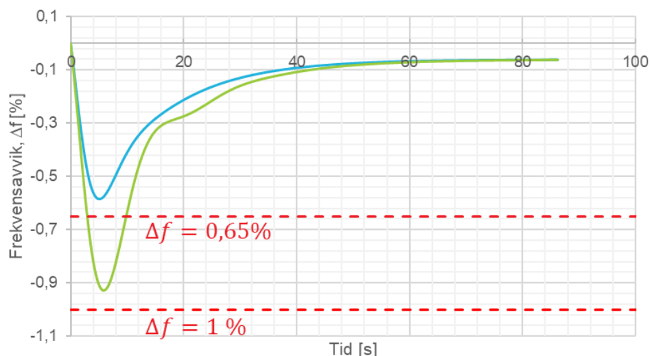
FIGUR 13-10: FREKVENSRRESPONS I TIDSPLANET VED 1 % LASTPÅSLAG REFERERT P_{maks} , VED P_{sett} = 85 \% \cdot P_{maks} OG 2 % STATISK. DE RØDE STIPLEDE LINJENE REPRERENTERER KRAVENE TIL MAKSIMALT TRANSIENT FREKVENSAVVIK. GRØNN (TYPE B OG C) OG BLÅ KURVER (TYPE D) ER EKSEMPLER PÅ FREKVENSFORLØP ETTER ET LASTSPRANG PÅ EGET OHMSK NETT.
