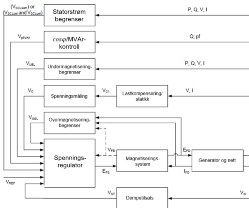
FIGUR 13-14: PRINSIPELL VIRKEMÅTE TIL SPENNINGSREGULATOREN FOR EN SYNKRON PRODUKSJONSENHET [11]. NB; MERK AT BLOKEDIAGRAMMET KUN VISER SPENNINGSINNGANG TIL DEMPETILSATS. DEMPETILSATS SKAL OGSÅ BENYTTET TURTALL IHT. KRAV I KAPITTEL 12.5.6.
