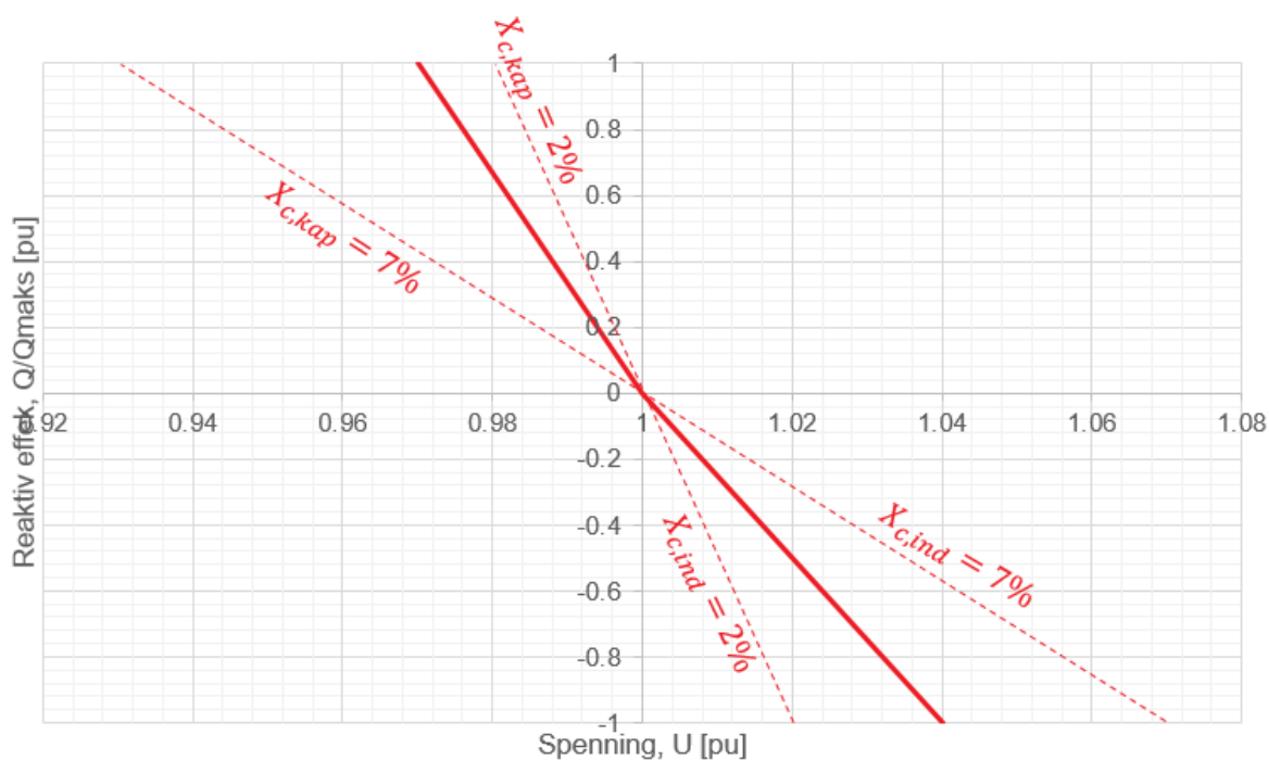
FIGUR 18-5: REAKTIV EFFEKT SOM FUNKSJON AV SPENNING I SPENNINGREGULERINGSMODUS FOR HVDC-SYSTEMET.
