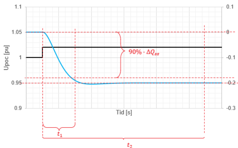
FIGUR 19-6: ILLUSTRASJON AV PRØVER FOR DOKUMENTASJON AV KRAV TIL UTREGULERINGSTID AV SPENNINGSREFERANSESTEG I POSITIV RETNING FOR HVDC-SYSTEM
