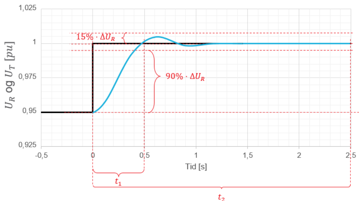
FIGUR 12-8: ILLUSTRASJON AV KRAV TIL UTREGULERINGSTID AV SPENNINGREFERANSESTEG I POSITIV RETNING FOR MAGNETISERINGSUTSTYR I LUKKET SLØYFE MED ÅPEN EFFEKTBRYTER FOR SYNKRONE PRODUKSJONSENHETER.
