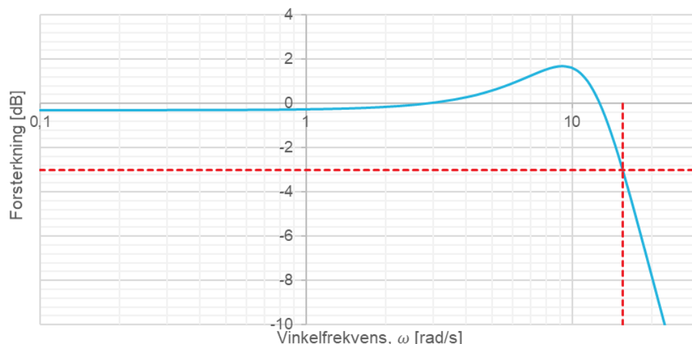
FIGUR 13-17: ILLUSTRASJON AV LUKKET SLØYFE-FORSTERKNING (BLÅ) FOR MAGNETISERINGSUTSTYR, MED BÅNDBREDDEN ILLUSTRERT (RØDSTIPEL)
