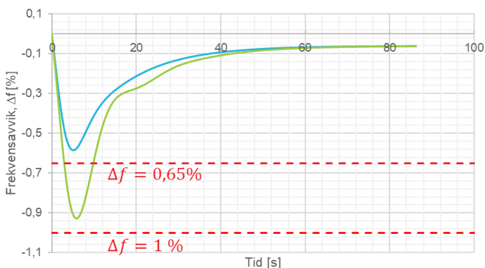
FIGUR 12-6: FREKVENSRSPONS I TIDSPLANET VED 1 % LASTPÅSLAG REFERERT P_{maks} , VED P_{sett} = 85 \% \cdot P_{maks} OG 2 % STATIKK. DE RØDE STIPELE LINJENE REPRERENTERER KRAVENE TIL MAKSIMALT TRANSIENT FREKVENSAVVIK. GRØNN (TYPE B OG C) OG BLÅ KURVER (TYPE D) ER EKSEMPLER PÅ FREKVENSFORLØP ETTER ET LASTSPRANG PÅ EGET OHMSK NETT.
