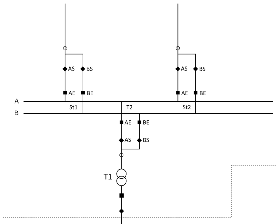
FIGUR 5-4: EKSEMPEL PÅ ENKELT BRYTERFELT PÅ SEKUNDÆRSIDE AV TRANSFORMATOR SOM TILKNYTTER EN ENKELT AVGANG
