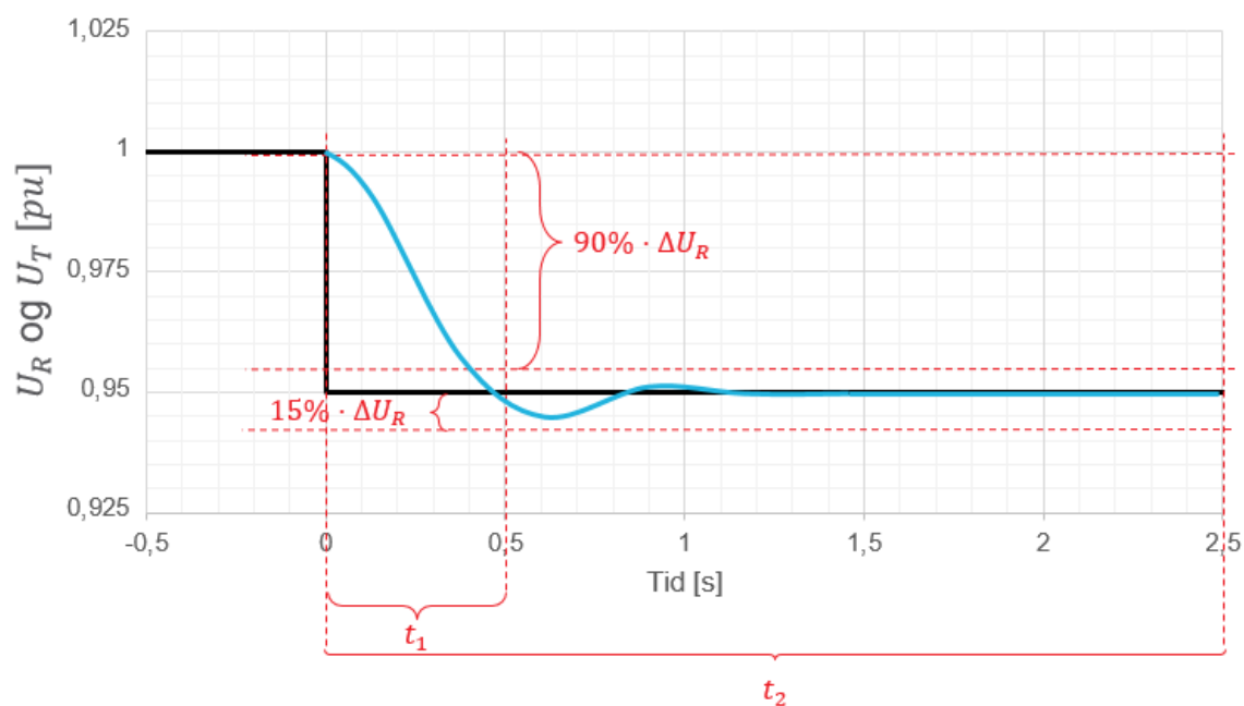
FIGUR 12-9: ILLUSTRASJON AV KRAV TIL UTREGULERINGSTID AV SPENNINGREFERANSESTEG I NEGATIV RETNING FOR MAGNETISERINGSUTSTYR I LUKKET SLØYFE MED ÅPEN EFFEKTBRYTER FOR SYNKRONE PRODUKSJONSENHETER.
