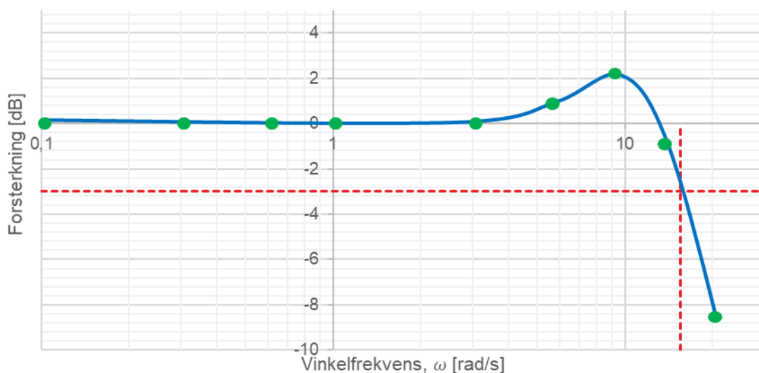
FIGUR 13-35: ILLUSTRASJON AV MAGNETISERINGSSYSTEMETS LUKKET SLØYFE-FORSTERKNING (BLÅ), MED BÅNDBREDDRE ILLUSTRERT (RØDSTIPELET). GRØNNE SIRKLER ILLUSTRERER DE TESTEDE PÅTRYKTE FREKVENSENE SOM ER TESTET.
