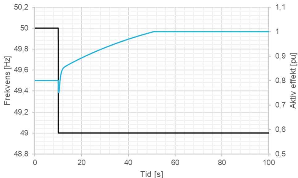
FIGUR 13-28: ILLUSTRASJON AV PRØVE AV AKTIV EFFEKTRESPONS (BLÅ) VED DETEKSJON AV SEPARATDRIFT VED HØY FREKVENSDRINGSFASTIGHET ( \Delta f/\Delta t , ROCOF) VED PÅTRYKKET FREKVENSRAMPE (SORT).
