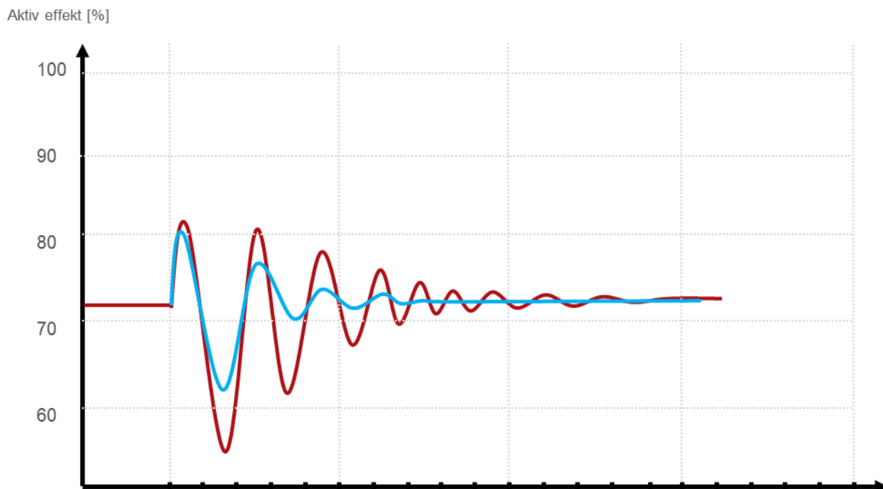
FIGUR 13-34: ILLUSTRASJON AV DEMPETILSATSENS EFFEKT PÅ EFFEKTPENDLINGER ETTER EN PÅTRYKKET SPENNINGSIMPULS. BLÅ VISER AKTIV EFFEKTRESPONS MED AKTIV DEMPETILSATS, OG RØD VISER AKTIV EFFEKTRESPONS UTEN DEMPETILSATS.
