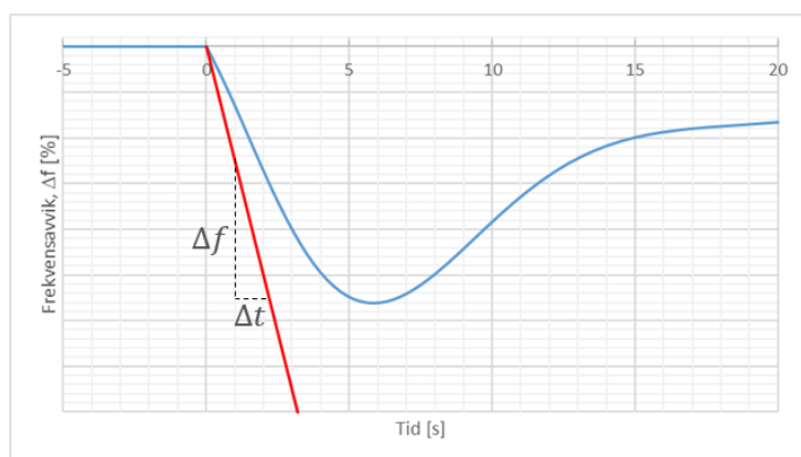
FIGUR 12-3: ILLUSTRASJON AV KRAV TIL FREKVENSDRINGSFASTIGHET. DERSOM FREKVENSFORLØPET ER OVER DEN RØDE LINJEN, SOM FALLER MED EN FREKVENSDRINGSFASTIGHET PÅ \frac{\Delta f}{\Delta t} = 1,5 \text{ Hz/s} , SKAL PRODUKSJONSENHETEN OPERERE NORMALT.
