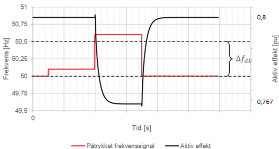
FIGUR 19-4: ILLUSTRASJON AV PRØVE FOR AKTIV EFFEKTRRESPONS (SORT) VED PÅTRYKKET FREKVENNSTEG(RØD) MED AKTIVE DØDBÅND (SORT STIPLET LINJE).
