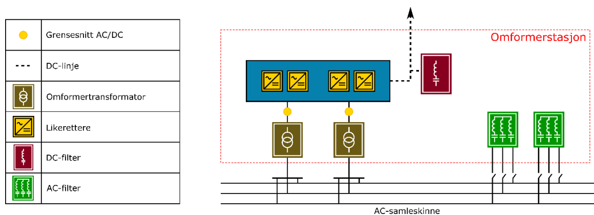
FIGUR 17-1: EKSEMPEL PÅ KOMPONENTER SOM KAN INNGÅ I EN OMFORMERSTASJON
