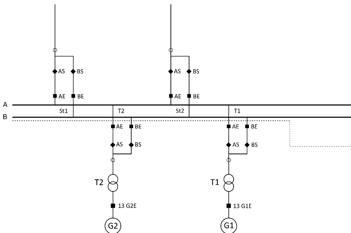
FIGUR 5-2: EKSEMPEL PÅ STASJONSLØSNING MED HØY FLEKSIBILITET FOR LUFTISOLERT ANLEGG; AB SAMLESKINNE, DOBLE EFFEKTBRYTEERE OG ENKLE STRØMTRANSFORMATORER
