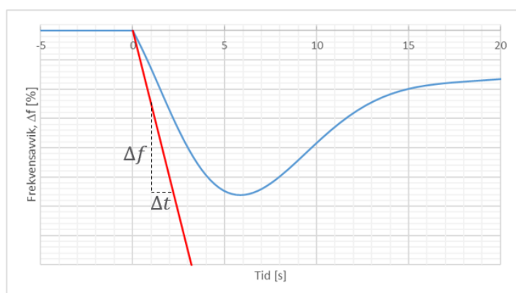
FIGUR 18-1: ILLUSTRASJON AV KRAV TIL FREKVENSEDRINGSHASTIGHET. DERSOM FREKVENSFORLØPET ER OVER DEN RØDE LINJEN, SOM FALLER MED EN FREKVENSEDRINGSHASTIGHET PÅ \frac{\Delta f}{\Delta t} = 2,5 Hz/s, SKAL HVDC-SYSTEMET KUNNE FORBLI TILKOBLET AC-NETTET.
