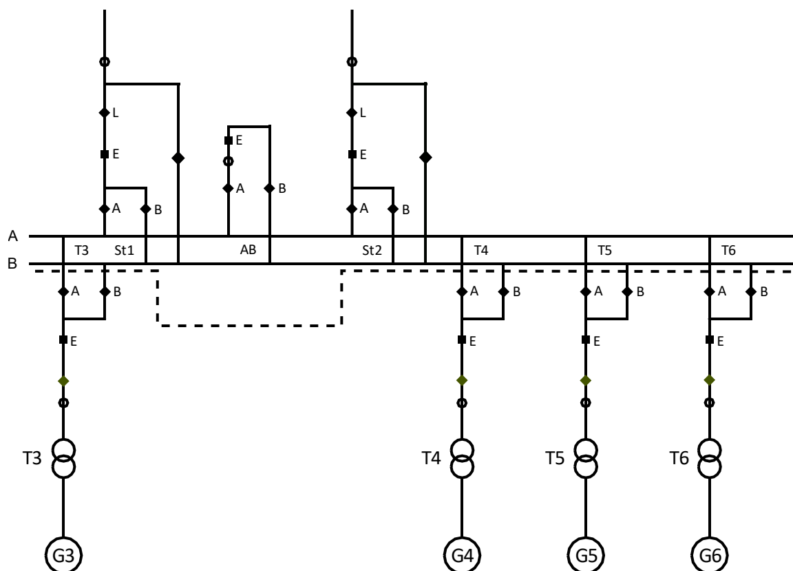
FIGUR 5-3: EKSEMPEL PÅ STASJONSLØSNING MED HØY FLEKSIBILITET; AB SAMLESKINNE, ENKLE EFFEKTBRYTEERE, ENKLE STRØMTRANSFORMATORER OG LEDNINGSFELT MED FORBIKOBLINGSMULIGHET.
