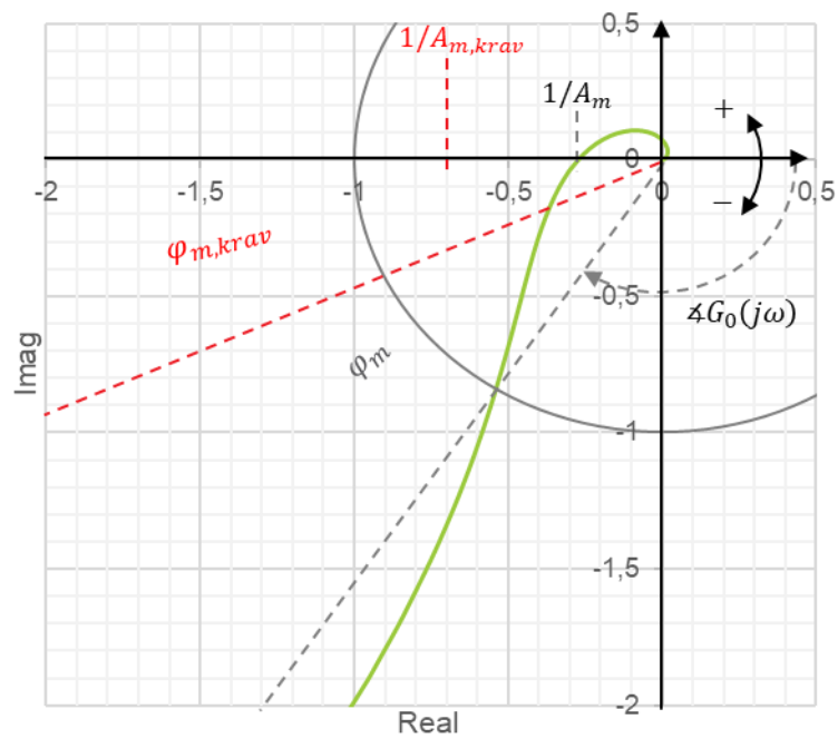
FIGUR 13-8: ILLUSTRASJON AV FREKVENSPÅNRESPONSEN (GRØNN) TIL G_o(s) , REF. LIGNING 13-1, I ET NYQUIST-DIAGRAM, HVILKET UTTRYKKER STABILITETEN TIL SYSTEMET. RØDSTIPLEDE LINJER INDIKERER KRAVENE TIL STABILITETSMARGIN. GRÅSTIPLEDE ER FAKTISK STABILITETSMARGIN.
