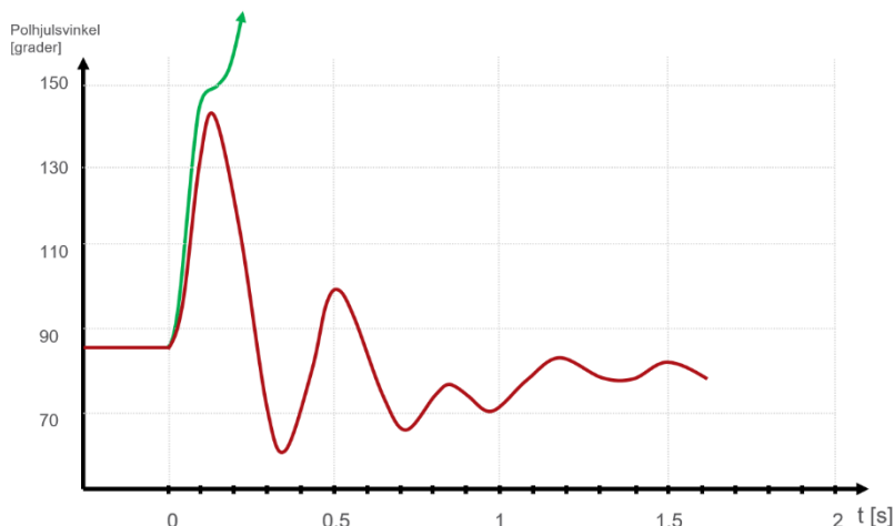
FIGUR 13-4: TYPISK TIDSFØRSLØP FOR ROTORVINKEL I TILKNYTNINGSPUNKT NÅR SYNKRONISME MOT NETTET BEHOLDRES (RØD) OG TAPES (GRØNN).
