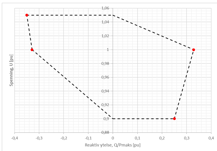
FIGUR 19-2: REAKTIV YTELSE FOR ET HVDC-SYSTEM VED VARIERENDE SPENNING, I U - Q/P_{maks} -PROFIL. RØDE PUNKTER ANGR VERDIENE SOM SKAL DOKUMENTERES.
