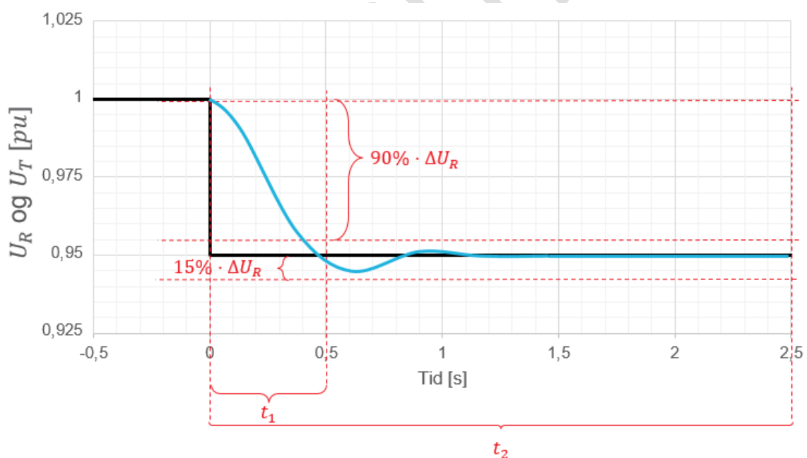
FIGUR 12-9: ILLUSTRASJON AV KRAV TIL UTREGULERINGSTID AV SPENNINGREFERANSESTEG I NEGATIV RETNING FOR MAGNETISERINGSUTSTYR I LUKKET SLØYFE MED ÅPEN EFFEKTBYTER FOR SYNKRONE PRODUKSJONSENHETER.
