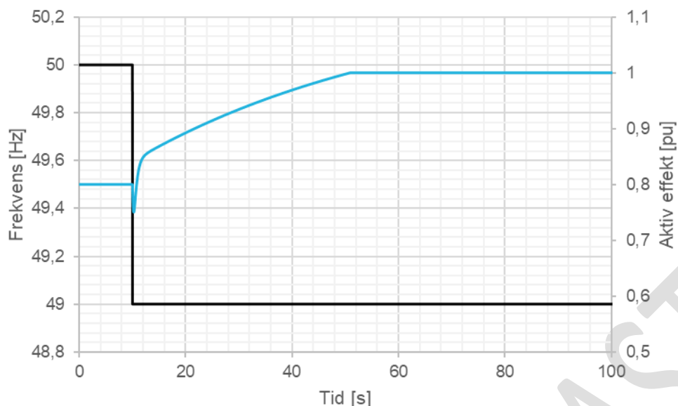
FIGUR 13-28: ILLUSTRASJON AV PRØVE AV AKTIV EFFEKTRESPONS (BLÅ) VED DETEKSJON AV SEPARATDRIFT VED HØY FREKVENSENDRINGSFASTIGHET ( \Delta f / \Delta t , ROCOF) VED PÅTRYKKET FREKVENSRAMPE (SORT).
