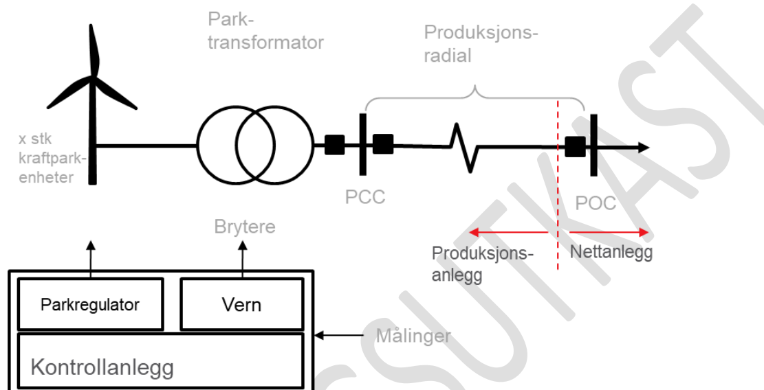
FIGUR 14-1: ILLUSTRASJON AV HOVEDKOMPONENTER I EN KRAFTPARK, HER VED EN VINDPARK, MED NOTASJONER. RØD STIPLET LINJE INDIKERER SKILLET MELLOM HVOR DET STILLES KRAV I DEL II NETTANLEGG OG DEL IV PRODUKSJONSENHETER.
