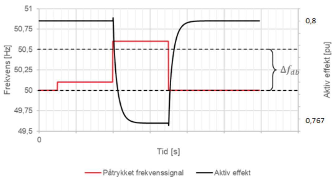
FIGUR 19-4 ILLUSTRASJON AV PRØVE FOR AKTIV EFFEKTPRESPONS (SORT) VED PÅTRYKKET FREKVENNSTEG (RØD) MED AKTIVE DØDBÅND (SORT STIPLET LINJE).
