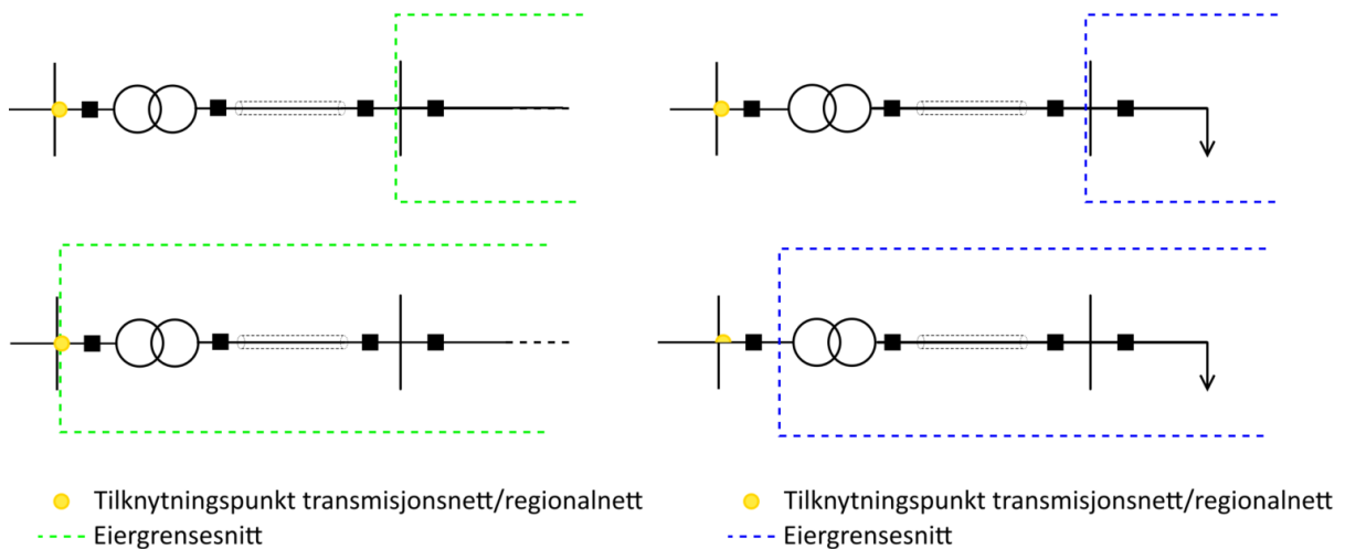
FIGUR 10-1 TILKOBLINGSPUNKT KAN VÆRE PÅ LAVSPENTSIDE AV TRANSFORMATOR TILKNYTTET REGIONAL ELLER TRANSMISJONSNETT, VED EIERGRENSESNIITT. MENS DERSOM TILKNYTNING VIA TRANSFORMATOR, VIL REFERANSE FOR TILKNYTNINGSPUNKTET VIL ALLTID VÆRE PÅ HØYSPENTSIDE AV TRANSFORMATOREN.
