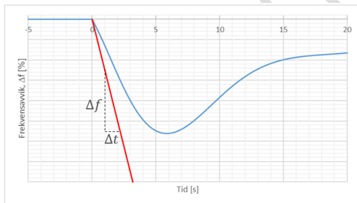
FIGUR 12-3: ILLUSTRASJON AV KRAV TIL FREKVENSDRINGSFASTIGHET. DERSOM FREKVENSFORLØPET ER OVER DEN RØDE LINJEN, SOM FALLER MED EN FREKVENSDRINGSFASTIGHET \text{PÅ} \frac{\Delta f}{\Delta t} = 1,5 \text{ Hz/s} , SKAL PRODUKSJONSENHETEN OPERERE NORMALT.
