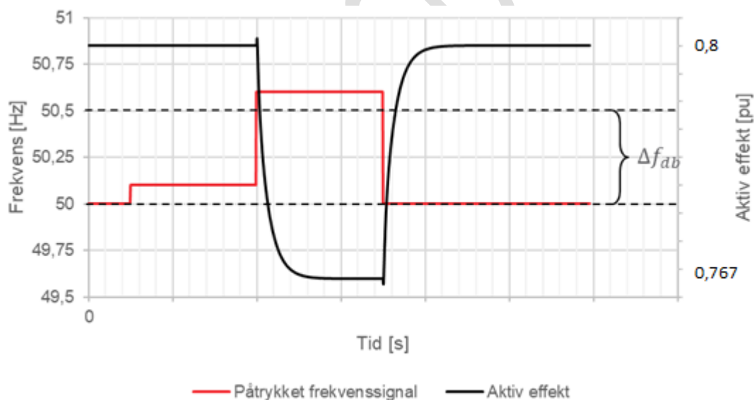
FIGUR 13-25: ILLUSTRASJON AV PRØVE FOR AKTIV EFFEKTRESPONS (SORT) VED PÅTRYKKET FREKVENNSTEG(RØD) MED AKTIVE DØDBÅND (SORT STIPLET LINJE).
