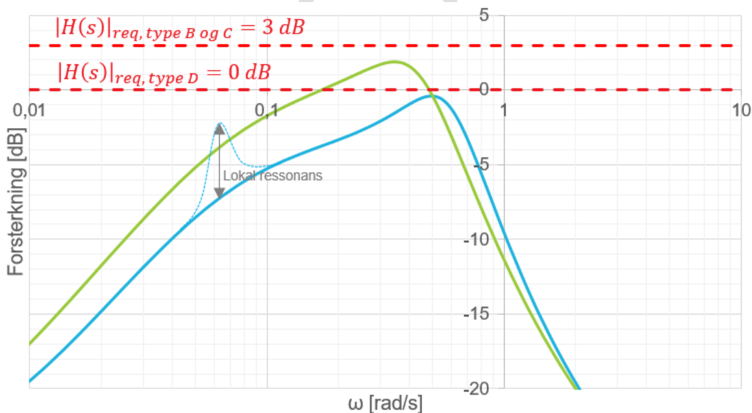
FIGUR 13-11: FREKVENSRSPONS ILLUSTRERT I FREKVENSPANET VED 1 % LASTPÅSLAG REFERERT P_{maks} , VED P_{sett} = 0,85 \cdot P_{maks} OG 2 % STATIKK. DE RØDE STIPELE LINJENE REPRERENTERER KRAVENE TIL MAKSIMALT TRANSIENT FREKVENSAVVIK. GRØNN (TYPE B OG C) OG BLÅ KURVER (TYPE D) ER EKSEMPLER PÅ FREKVENSFORLØP ETTER ET LASTSPRANG PÅ EGET OHMSK NETT.
