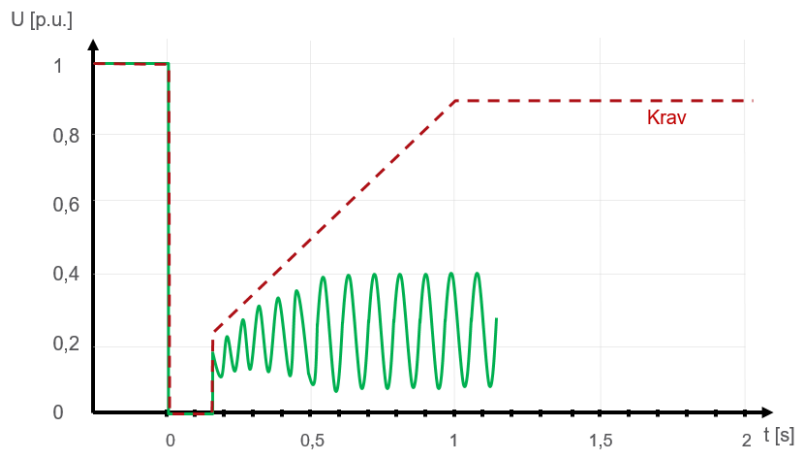
FIGUR 13-3: TYPISK TIDSFORLØP FOR SPENNING I TILKNYTNINGSPUNK NÅR SYNKRONISME MOT NETTET TAPES VED FEILKLARERINGS-TID > CCT, NÅR SPENNINGEN ETTER FEIL LIGGER UNDER KRAVKURVEN.
