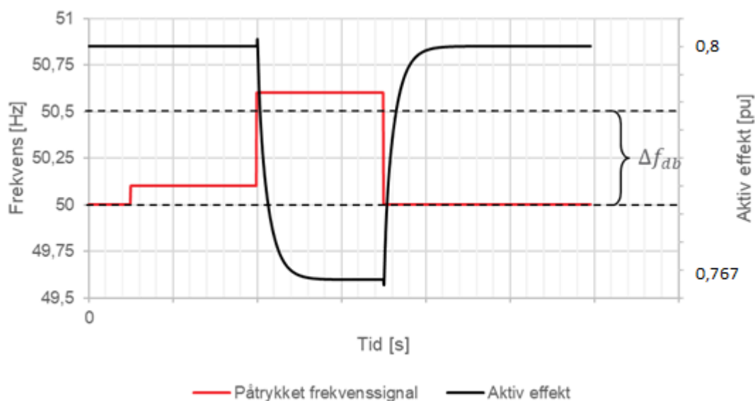
FIGUR 16-5: ILLUSTRASJON AV PRØVE FOR AKTIV EFFEKTTRESPONS (SORT) VED PÅTRYKKET FREKVENSTEG (RØD) MED AKTIVE DØDBÅND (SORT STIPLLET LINJE).
