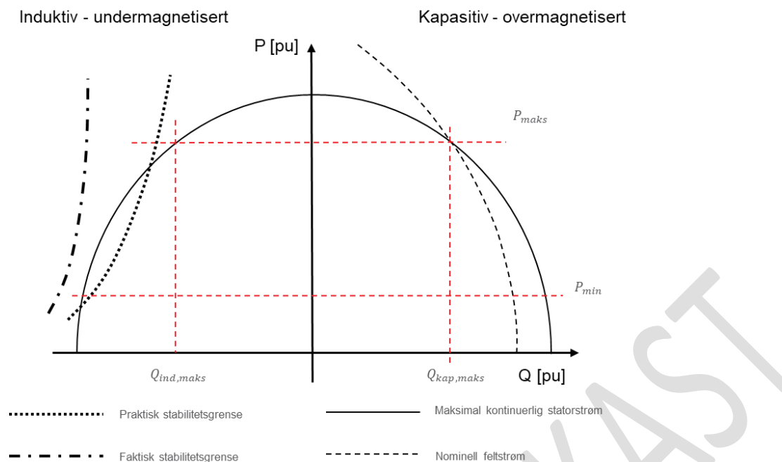
FIGUR 12-7: DRIFSDIAGRAMMET TIL EN TYPISK SYNKROGENERATOR
