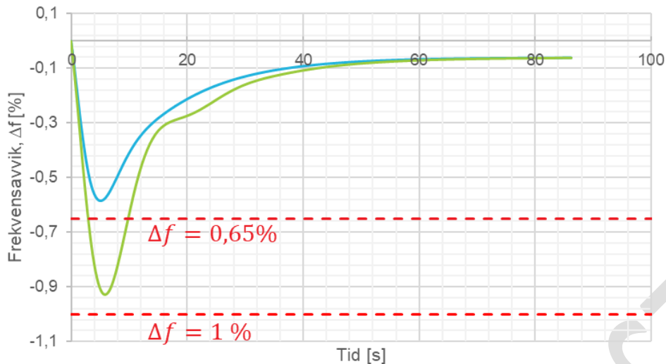
FIGUR 13-10: FREKVENSRSPONS I TIDSPLANET VED 1 % LASTPÅSLAG REFERERT P_{maks} , VED P_{sett} = 85 \% \cdot P_{maks} OG 2 % STATIKK. DE RØDE STIPELE LINJENE REPRERENTERER KRAVENE TIL MAKSIMALT TRANSIENT FREKVENSAVVIK. GRØNN (TYPE B OG C) OG BLÅ KURVER (TYPE D) ER EKSEMPLER PÅ FREKVENSFORLØP ETTER ET LASTSPRANG PÅ EGET OHMSK NETT.
