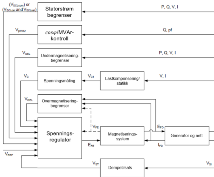
FIGUR 13-14: PRINSIPELL VIRKEMÅTE TIL SPENNINGSREGULATOREN FOR EN SYNKRON PRODUKSJONSENHET [11]. NB; MERK AT BLOKDDIAGRAMMET KUN VISER SPENNINGSINNGANG TIL DEMPETILSATS. DEMPETILSATS SKAL OGSÅ BENYTTE TURTALL IHT. KRAV I KAPITTEL 12.5.6.
