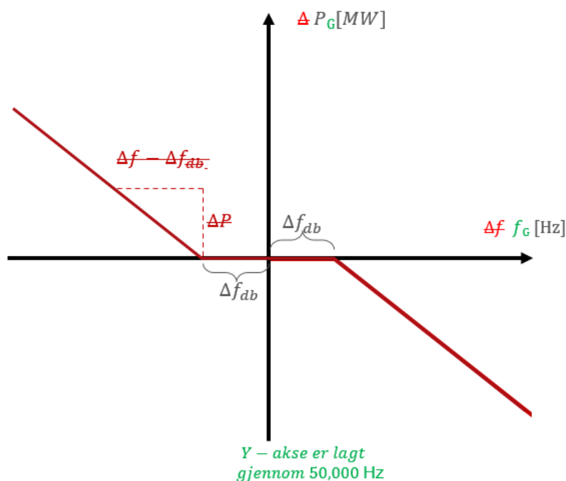
FIGUR 12-4: REGULATORRESPONS SOM FUNKSJON AV FREKVENSI I FREKVENSRULERINGSMODUS FOR SYNKRONE PRODUKSJONSENHETER.
