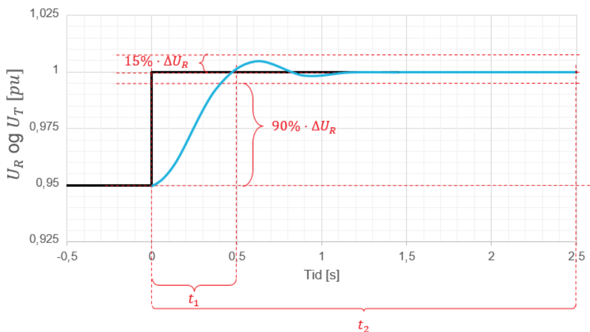
FIGUR 12-8: ILLUSTRASJON AV KRAV TIL UTREGULERINGSTID AV SPENNINGREFERANSESTEG I POSITIV RETNING FOR MAGNETISERINGSUTSTYR I LUKKET SLØYFE MED ÅPEN EFFEKTBYTER FOR SYNKRONE PRODUKSJONSENHETER.
