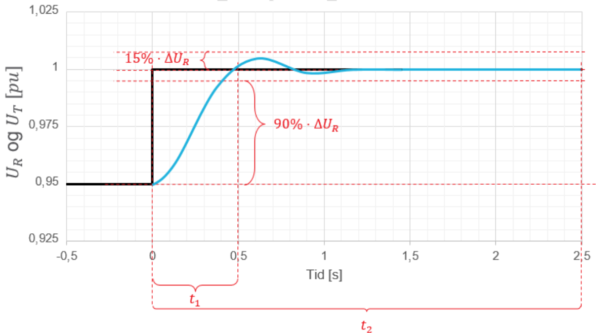
FIGUR 13-15: ILLUSTRASJON AV KRAV TIL UTREGULERINGSTID AV SPENNINGSREFERANSESTEG I POSITIV RETNING FOR MAGNETISERINGSUTSTYR I LUKKET SLØYFE MED ÅPEN EFFEKTBRUYER FOR SYNKRONE PRODUKSJONSENHETER.
