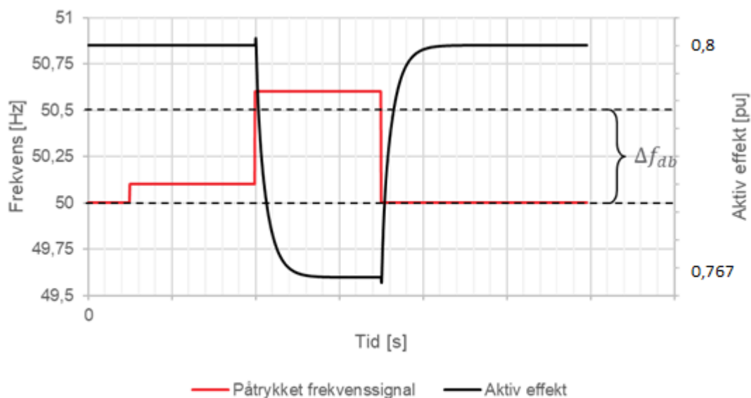
FIGUR 16-5: ILLUSTRASJON AV PRØVE FOR AKTIV EFFEKTRESPONS (SORT) VED PÅTRYKKET FREKVENSSTEG(RØD) MED AKTIVE DØDBÅND (SORT STIPLET LINJE).
