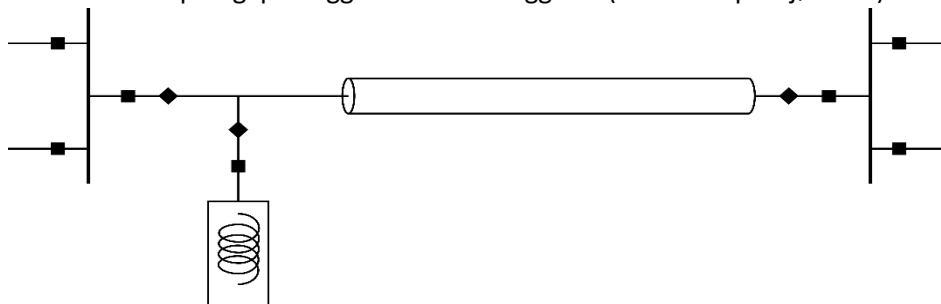
FIGUR 5-6: EKSEMPEL PÅ T-AVGRENING MED BRYTER TIL KOMPENSERINGSANLEGG - BEHOVSPRØVD FLEKSIBILITET I FORHOLD TIL AT KOMPENSERINGSANLEGGET IKKE KAN VÆRE TIL NYTTE FOR KRAFTSYSTEMET NÅR SJØKABEL IKKE ER I DRIFT
