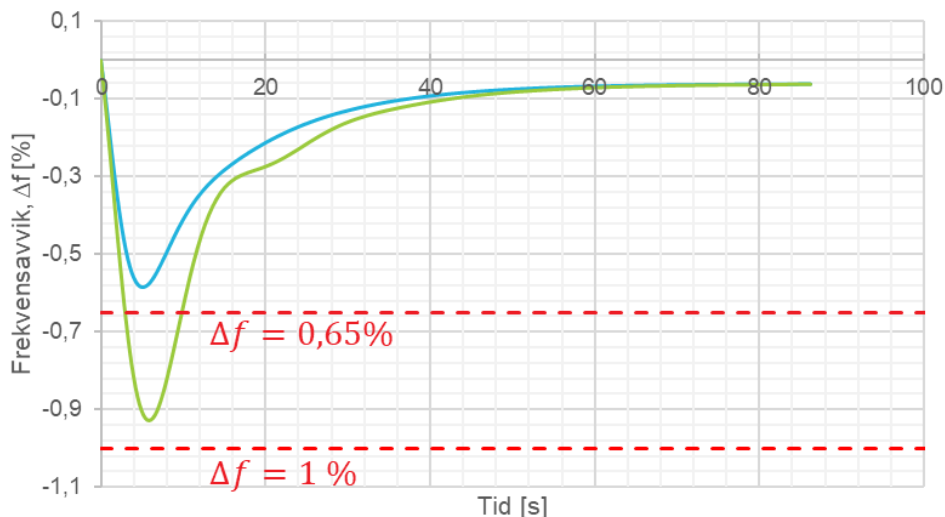
FIGUR 13-10: FREKVENSRSPONS I TIDSPLANET VED 1 % LASTPÅSLAG REFERERT P_{maks} , VED P_{sett} = 85\% \cdot P_{maks} OG 2 % STATISK. DE RØDE STIPLEDE LINJENE REPRERENTERER KRAVENE TIL MAKSIMALT TRANSIENT FREKVENSAVVIK. GRØNN (TYPE B OG C) OG BLÅ KURVER (TYPE D) ER EKSEMPLER PÅ FREKVENSFØRLØP ETTER ET LASTSPRANG PÅ EGET OHMSK NETT.
