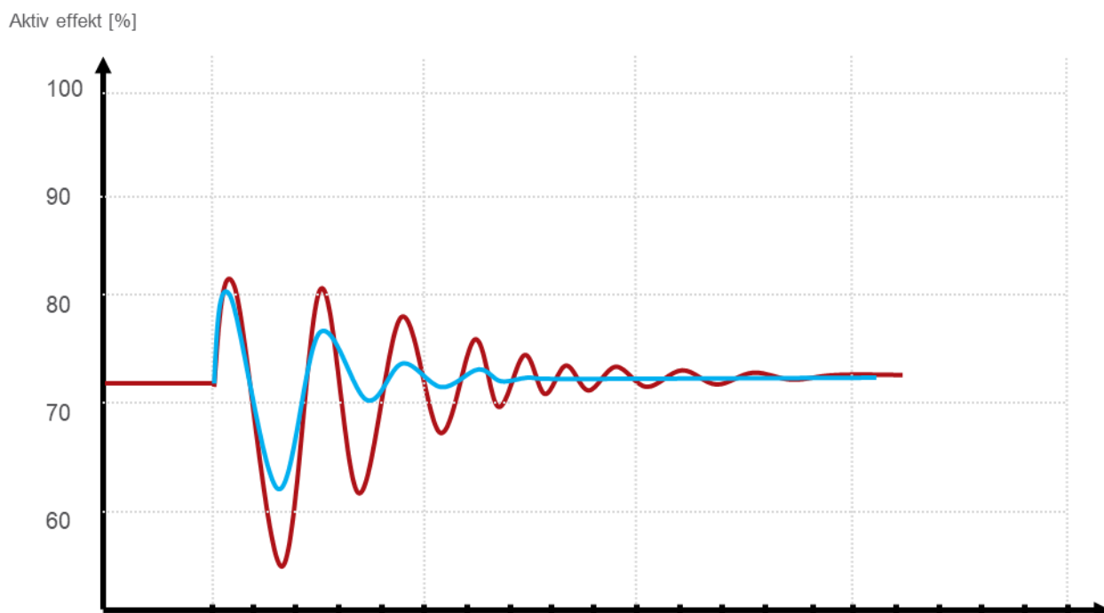
FIGUR 13-33: ILLUSTRASJON AV DEMPETILSATSENS EFFEKT PÅ EFFEKTPENDLINGER ETTER EN PÅTRYKKET SPENNINGSIMPULS. BLÅ VISER AKTIV EFFEKTRESPONS MED AKTIV DEMPETILSAT, OG RØD VISER AKTIV EFFEKTRESPONS UTEN DEMPETILSAT.
