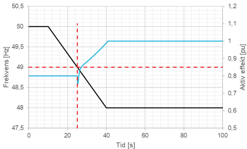
FIGUR 13-27: ILLUSTRASJON AV PRØVE AV AKTIV EFFEKTRESPONS (BLÅ) VED DETEKSJON AV SEPARATDRIFT VED FREKVENSTERSKEL VED PÅTRYKKET FREKVENSRAMPE (SORT). BLÅ KURVE VISER ENDRING I PARAMETERSETT VED FREKVENNS < 49 Hz.
