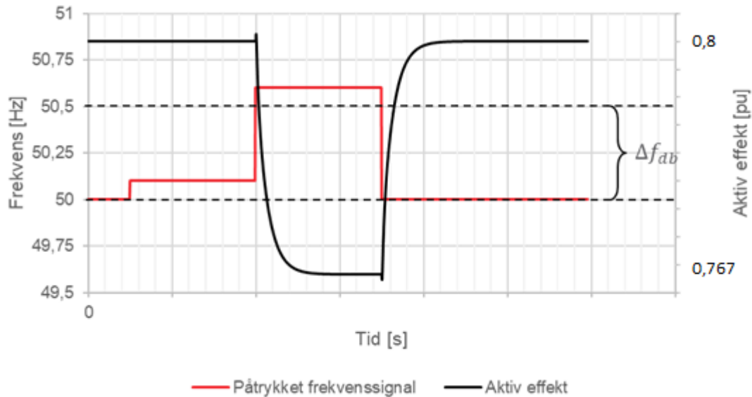
FIGUR 13-25: ILLUSTRASJON AV PRØVE FOR AKTIV EFFEKTRESPONS (SORT) VED PÅTRYKKET FREKVENSTEG (RØD) MED AKTIVE DØDBÅND (SORT STIPILET LINJE).
