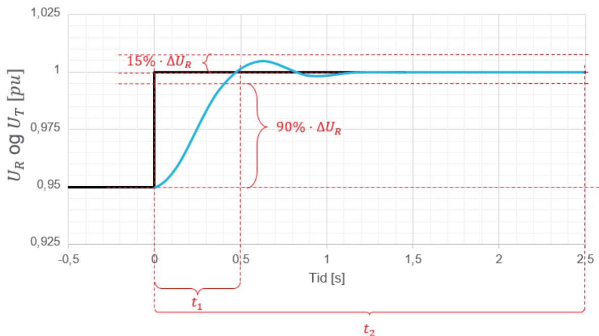
FIGUR 12-8: ILLUSTRASJON AV KRAV TIL UTREGULERINGSTID AV SPENNINGREFERANSESTEG I POSITIV RETNING FOR MAGNETISERINGSUTSTYR I LUKKET SLØYFE MED ÅPEN EFFEKTBRUYER FOR SYNKRONE PRODUKSJONSENHETER.
