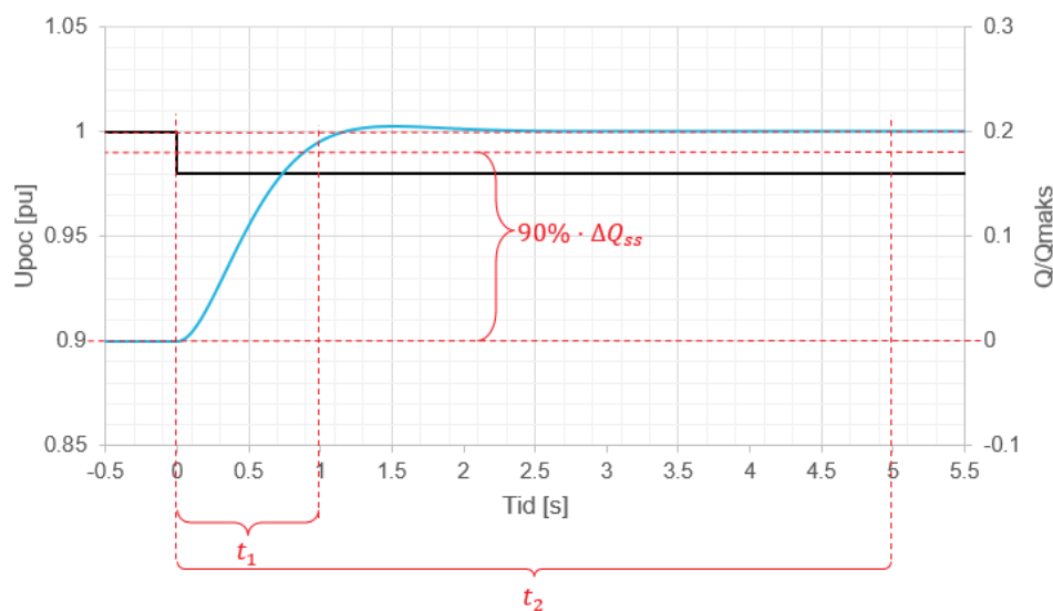
FIGUR 16-7: ILLUSTRASJON AV PRØVER FOR DOKUMENTASJON AV KRAV TIL UTREGULERINGSTID AV SPENNINGREFERANSESTEG I POSITIV RETNING FOR KRAFTPARK.
