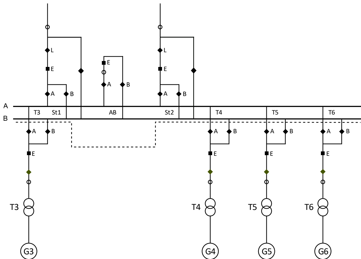
FIGUR 5-3: EKSEMPEL PÅ STASJONSLØSNING MED HØY FLEKSIBILITET; AB SAMLESKINNE, ENKLE EFFEKTBRYTERE, ENKLE STRØMTRANSFORMATORER OG LEDNINGSFELT MED FORBIKOBLINGSMULIGHET.
