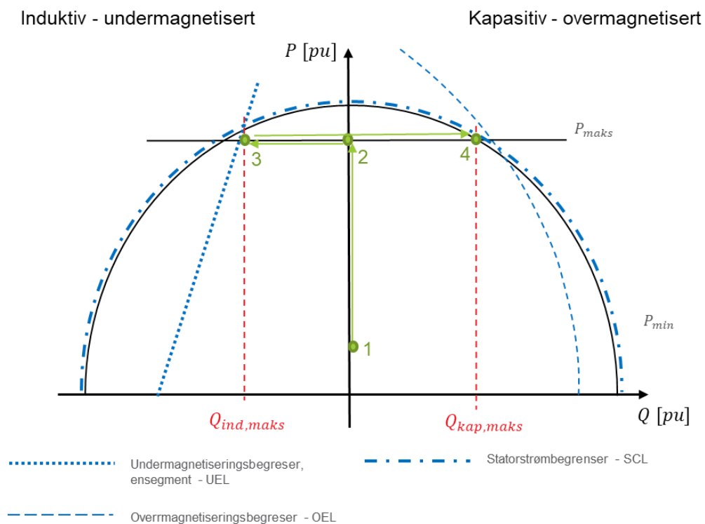
FIGUR 13-35: ILLUSTRASJON AV METODE FOR GJENNOMFØRING AV TEST AV REAKTIV YTELSE FOR SYNKRONE PRODUKSJONSENHETER. GRØNNE PUNKTER HENVISER TIL PUNKTLISTE OVER.
