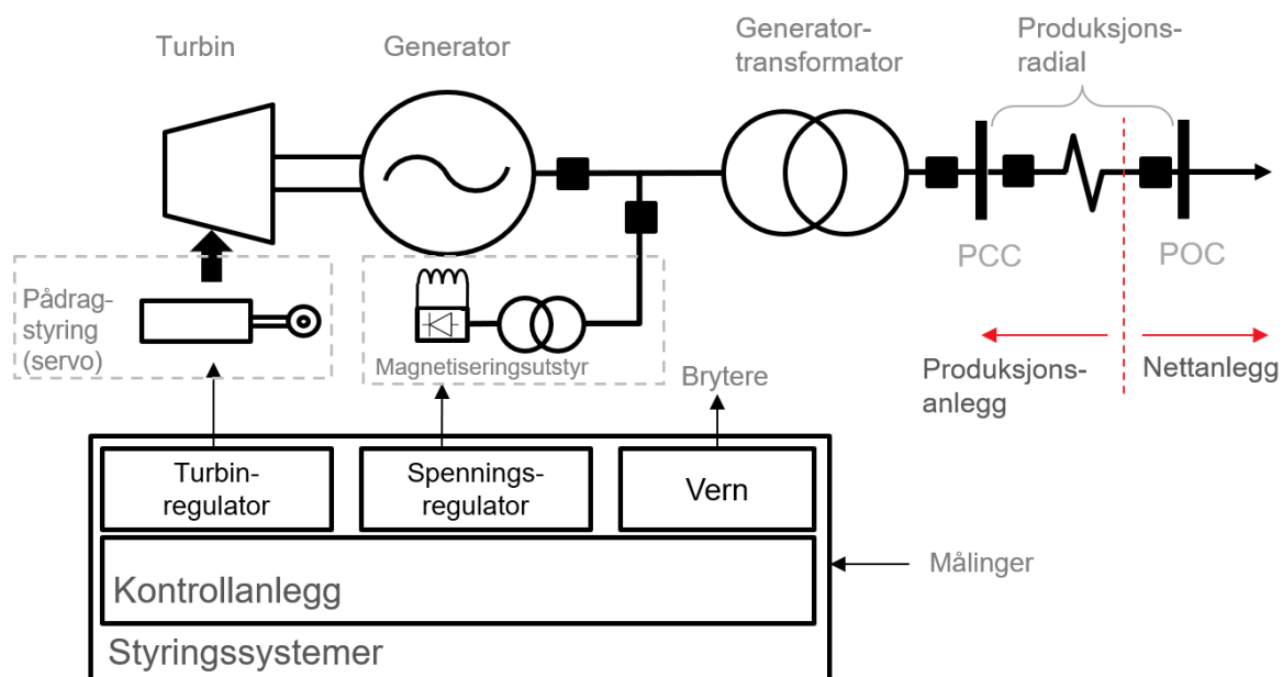
FIGUR 12-1: HOVEDKOMponenter I SYNKRONE PRODUKSJONSENHETER. RØD STIPILET LINJE INDIKERER SKILLET MELLOM HVOR DET STILLES KRAV I DEL II NETTANLEGG OG DEL IV PRODUKSJONSANLEGG.
