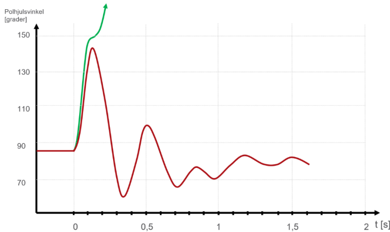
FIGUR 13-4: TYPISK TIDSFØRSLØP FOR ROTORVINKEL I TILKNYTNINGSPUNKT NÅR SYNKRONISME MOT NETTET BEHOLDES (RØD) OG TAPES (GRØNN).
