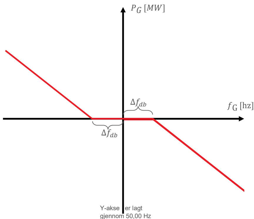
FIGUR 12-4: REGULATORRESPONS SOM FUNKSJON AV FREKVENSI I FREKVENSRGULERINGSMODUS FOR SYNKRONE PRODUKSJONSENHETER.
