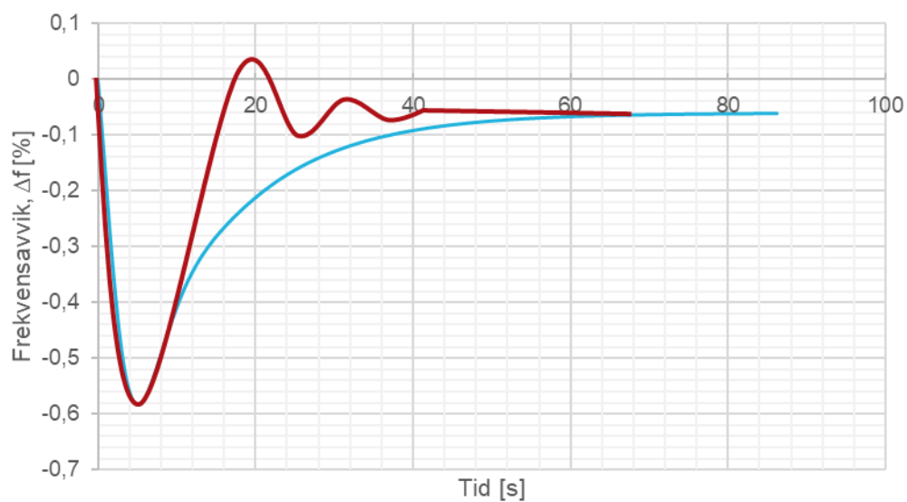
FIGUR 13-28: FREKVENS AVVIK, RESPONS I TIDSPLANET
