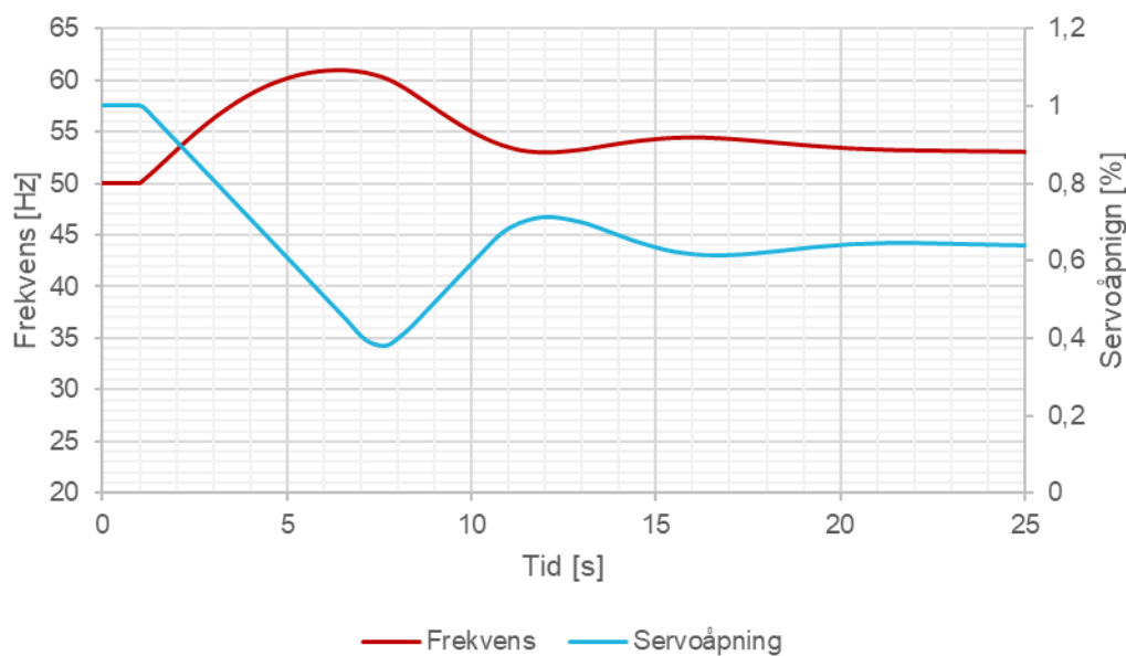
FIGUR 13-30: ILLUSTRASJON AV SIMULERING AV ET STORT LASTSPRANG HVOR ULINEARITETER ER DOMINERENDE, HER SYNLIG VED VENTILMETNING I OLJETRYKKANLEGG, SOM GIR KONSTANT ENDRINGSHASTIGHET PÅ SERVOÅPNING.
