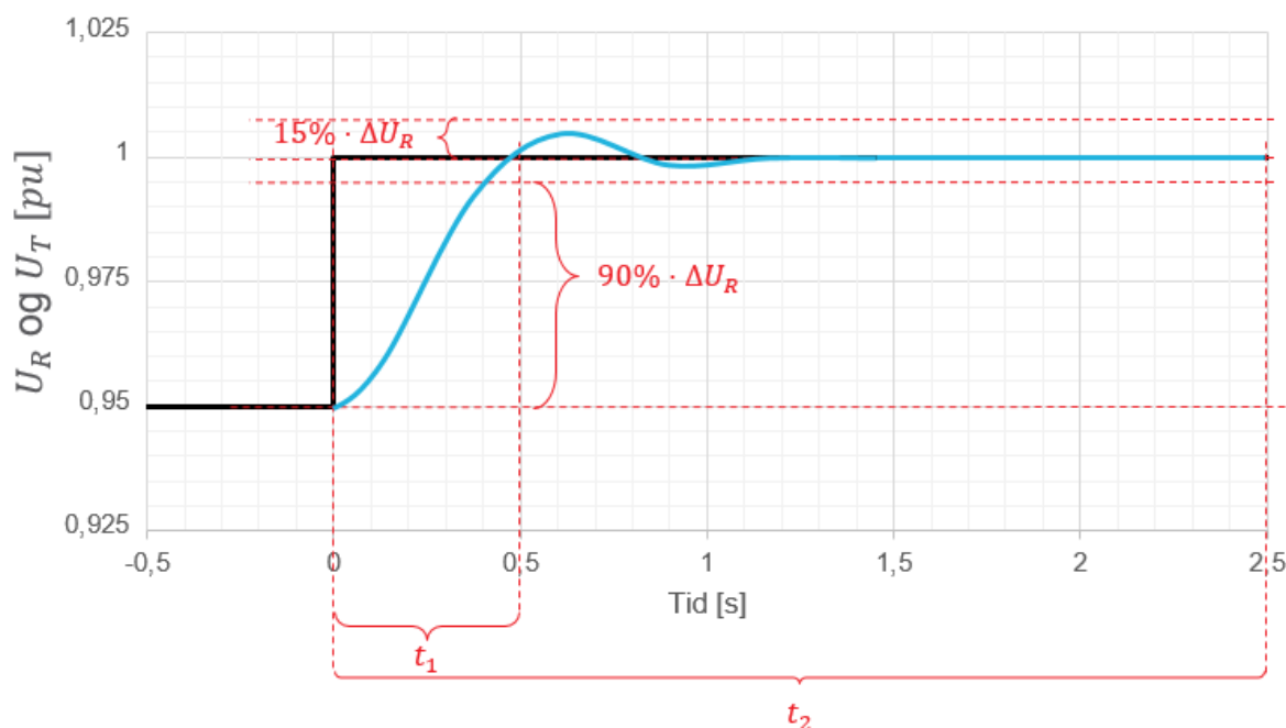
FIGUR 13-31: ILLUSTRASJON AV PRØVER FOR DOKUMENTASJON AV KRAV TIL UTREGULERINGS- TID AV SPENNINGREFERANSESTEG I POSITIV RETNING FOR MAGNETISERINGSUTSTYR MED ÅPNE GENERATORKLEMMER FOR SYNKRONE PRODUKSJONSENHETER.
