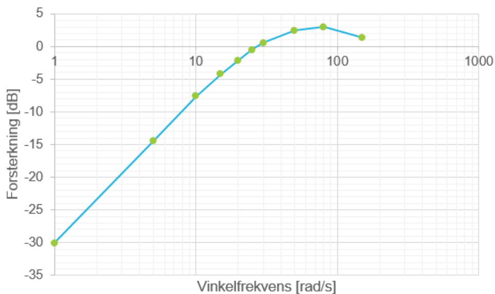
FIGUR 13-29: FORSTERKNING, DET REGULERTE SYSTEMETS EVNE TIL Å UNDERTRYKKE FORSTYRRELSER
