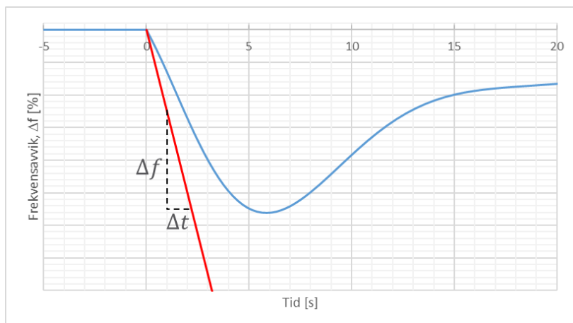
FIGUR 14-2: ILLUSTRASJON AV KRAV TIL FREKVENSDRINGSFASTHET. DERSOM FREKVENSFORLØPET ER OVER DEN RØDE LINJEN, SOM FALLER MED EN FREKVENSDRINGSFASTHET PÅ \frac{\Delta f}{\Delta t} = 1,5 \text{ Hz/s} , SKAL PRODUKSJONSENHETEN OPERERE NORMALT.
