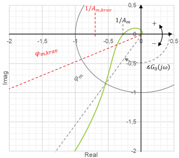
FIGUR 13-8: ILLUSTRASJON AV FREKVENSPÅNRESPONSEN (GRØNN) TIL G_o(s) , REF. LIGNING 13-1, I ET NYQUIST-DIAGRAM, HVILKET UTTRYKKER STABILITETEN TIL SYSTEMET. RØDSTIPELE LINJER INDIKERER KRAVENE TIL STABILITETSMARGIN. GRÅSTIPELE ER FAKTISK STABILITETSMARGIN.
