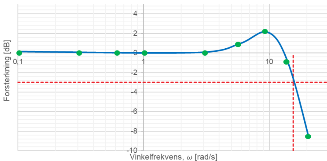
FIGUR 13-34: ILLUSTRASJON AV MAGNETISERINGSSYSTEMETS LUKKET SLØYFE-FORSTERKNING (BLÅ), MED BÅNDBREDDEN ILLUSTRERT (RØDSTIPEL). GRØNNE SIRKLER ILLUSTRERER DE TESTEDE PÅTRYKTE FREKVENSENE SOM ER TESTET.
