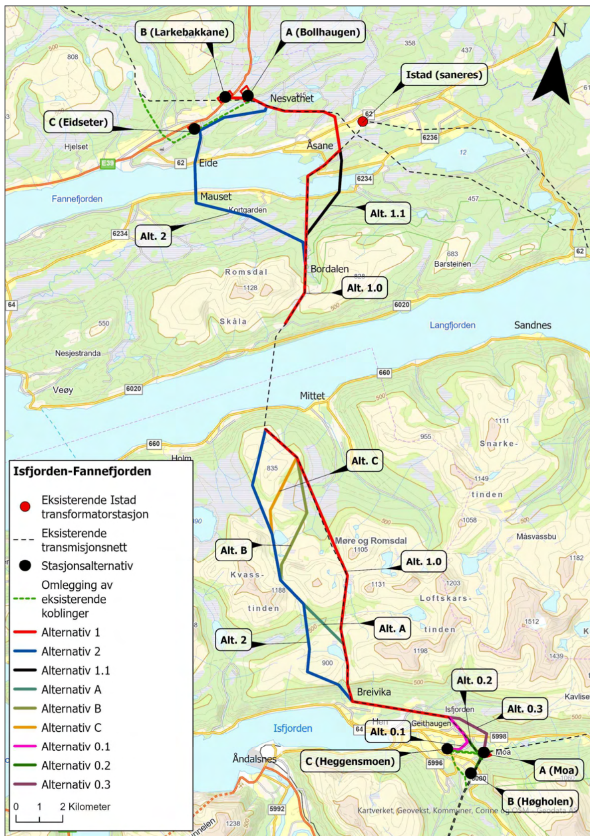
Figur 4 Meldte ledningstraséer mellom Fannefjorden og Isfjorden. Nytt spenn fra 2020 over Langfjorden gjenbrukes. Dagens traséer for 420 og 132 kV vist med stiplede strek. Innføring til stasjon i Isfjorden kan gjøres med noen variasjoner avhengig av stasjonens plassering, se kapittel 4.1.6.
