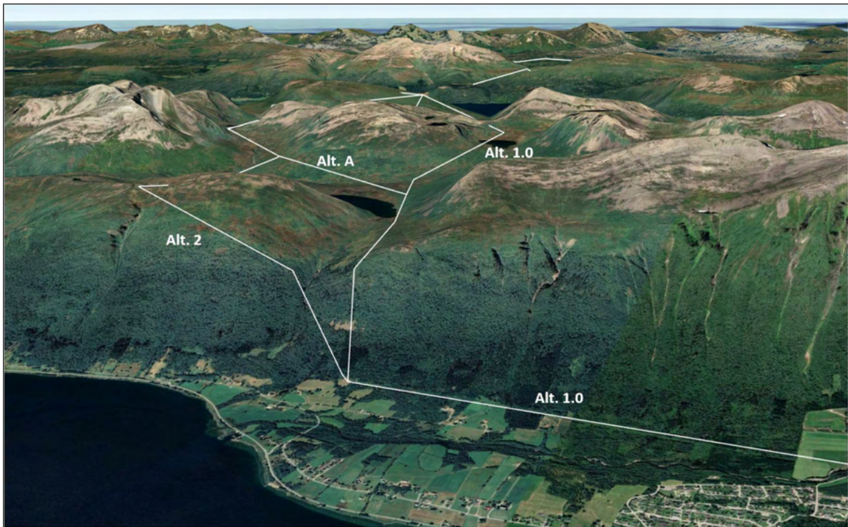
Figur 33 Ledningstraséene vist i terrenget. Dagens trasé ligger inne i alt 1.0, og synligheten av ny ledning vil bli noe tilsvarende, men med noe større master. Kilde :Google Earth.
