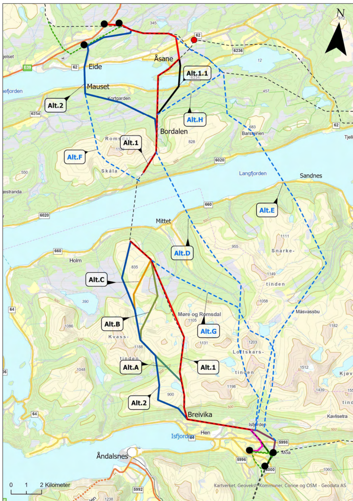
Figur 23 Forkastede alternativ med blå stiplede linje (D-G) og meldte traséer nummerert. Dagens traséer for 132 og 420 kV vist med stiplede svart linje.
