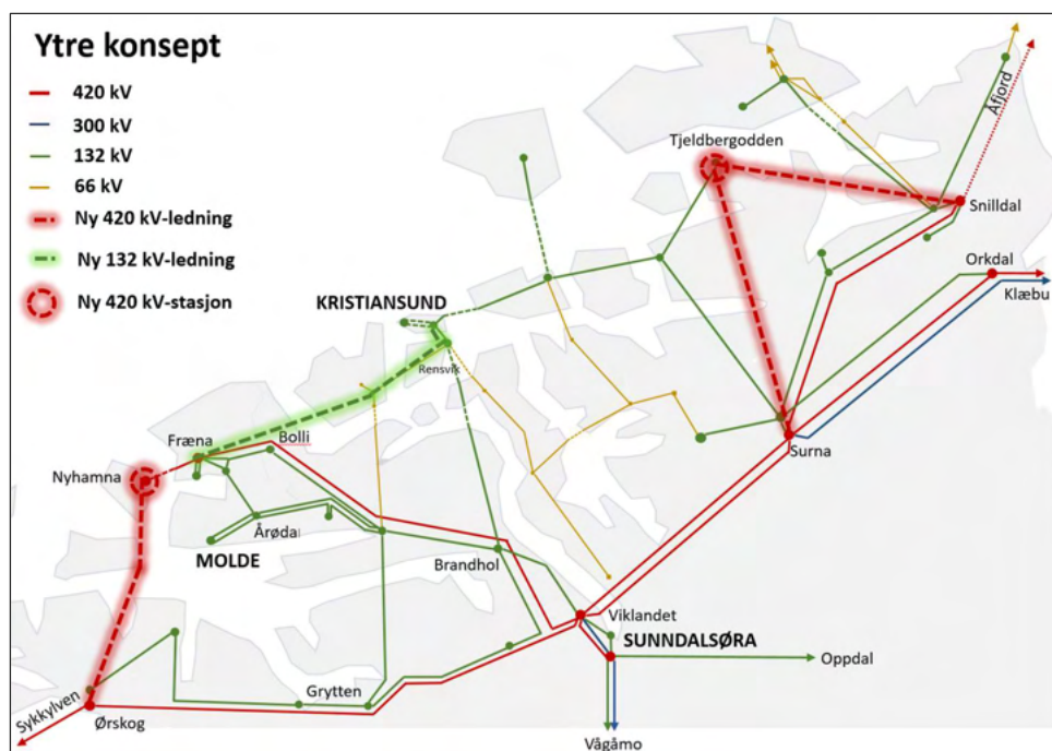
Figur 8: Ytre konsept er forkastet.
