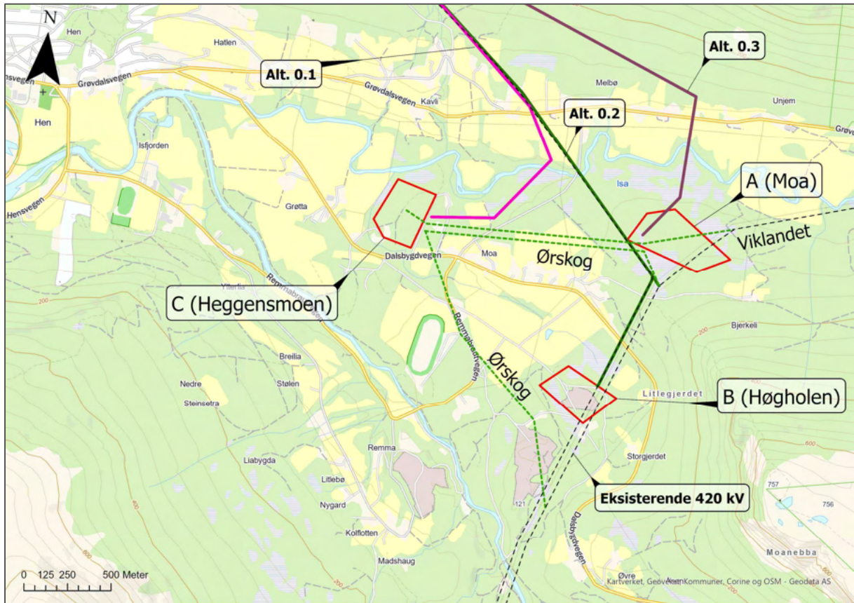
Figur 17 Alternativ C Heggensmoen med mulige løsninger for ledninger som foreslås utredet.
