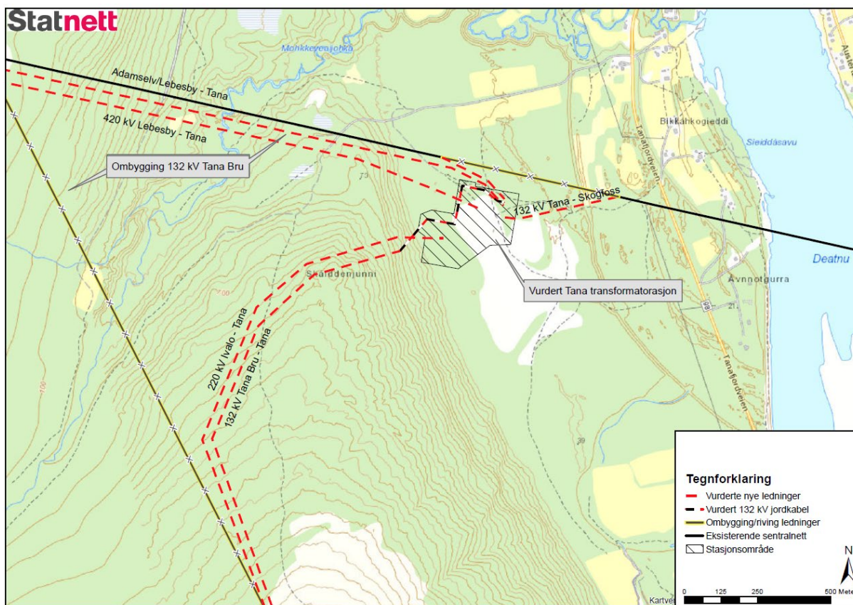
Figur 22: Kart som viser vurdert plassering av Tana transformatorstasjon med tilhørende omlegging av ledninger til stasjonen. Se også oversiktskart i figur 17 som viser omlegging av 220 kV til Ivalo.
