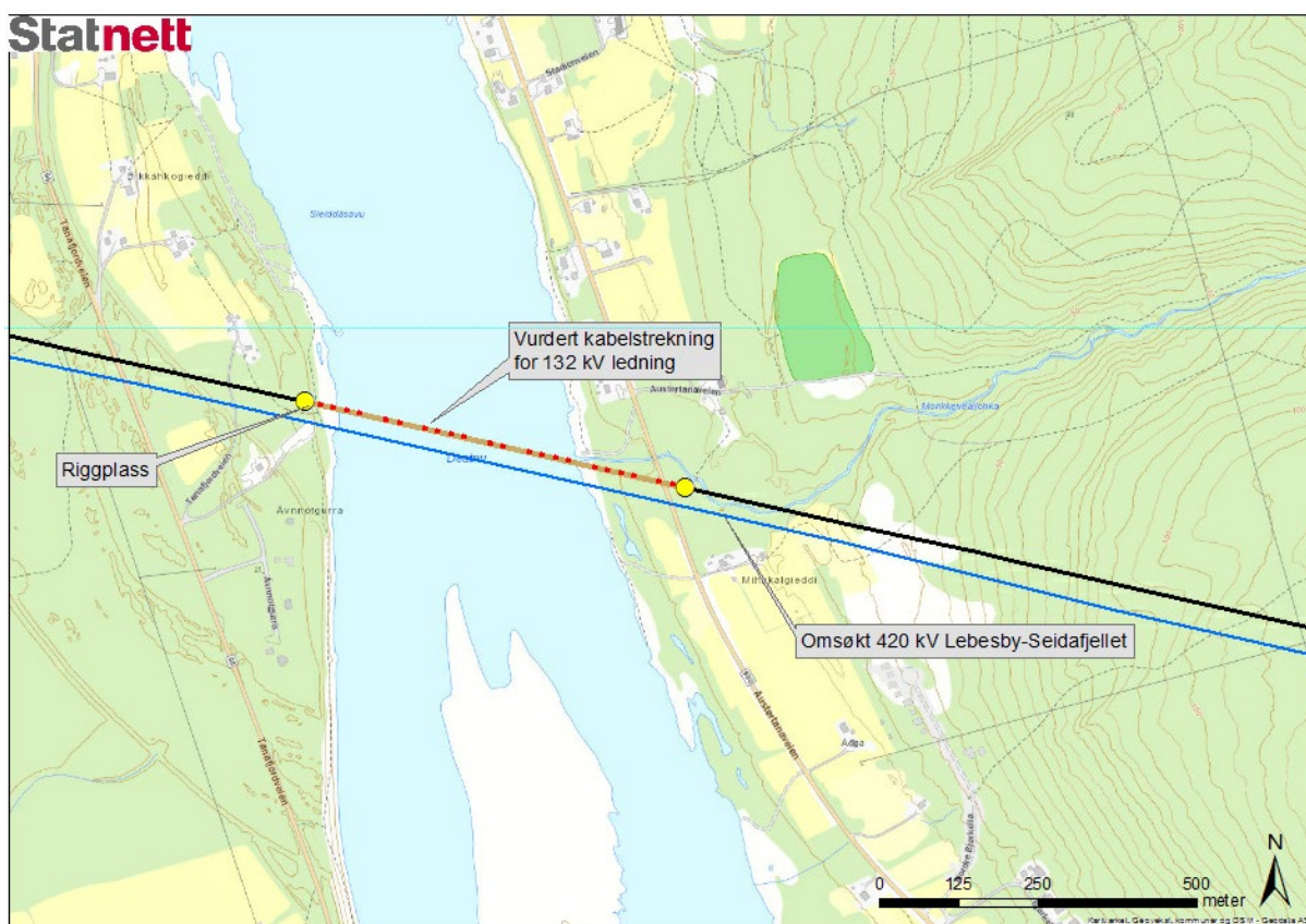
Figur 25: Kabel for 132 kV ledningen Adamselv-Varangerbotn ved kryssingen av Tana. Kartet viser også punkter for riggplasser på hver side av den vurderte kabelstrekningen.
