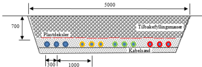
Figur 28: En prinsippskisse som viser tverrsnitt av en kabelgrøft med 4 stk 132 kV kabler.
