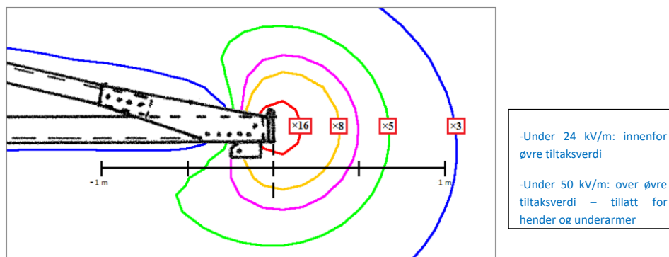
Figur 16: Beregnende forsterkningsfaktorer for E-felt ved traversspiss
