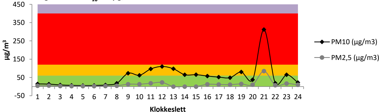
Figur 5-4 Timesmidler PM 10 og PM 2,5 for overskridelsesdøgn fredag 12.04.24. Fargeklassifiseringen for varslingsklassene basert på helsevirkninger gjelder for PM 10 (svart kurve).
