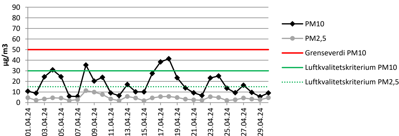
Figur 5-6 Døgnmidler PM 10 og PM 2,5 ved Rektorhaugen i april 2024, inkludert døgn grenseverdi for PM 10 på 50 µg/m 3 , og luftkvalitetskriteriene for døgnmidler PM 10 og PM 2,5 .
