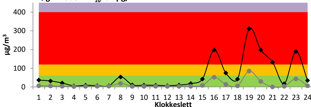
Figur 5-3 Timesmidler PM 10 og PM 2,5 for overskridelsesdøgn torsdag 11.04.24. Fargeklassifiseringen for varslingsklassene basert på helsevirkninger gjelder for PM 10 (svart kurve).
