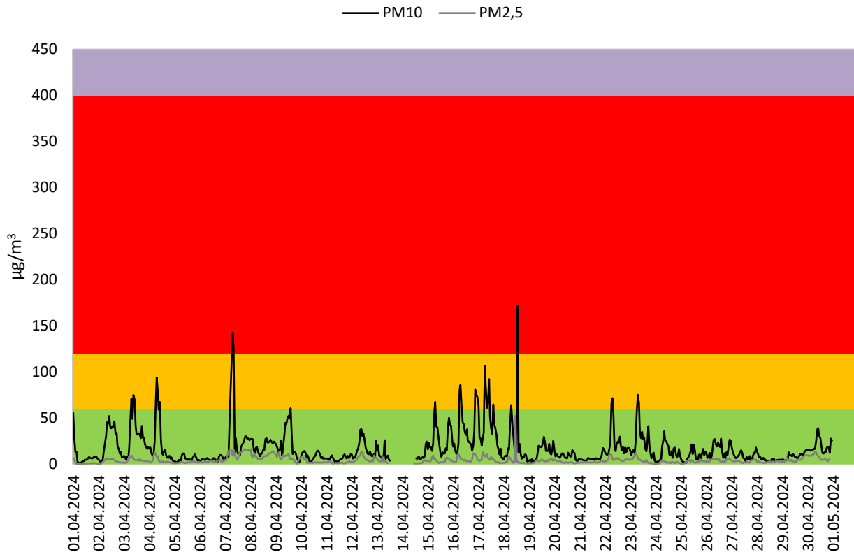
Figur 5-7 Timesmidler PM 10 og PM 2,5 ved Ulven i april 2024. Fargeklassifiseringen for varslingsklassene basert på helsevirkninger gjelder for PM 10 (svart linje). Grønn klasse: Liten eller ingen helserisiko, gul klasse: moderat helserisiko, rød klasse: betydelig helserisiko.
