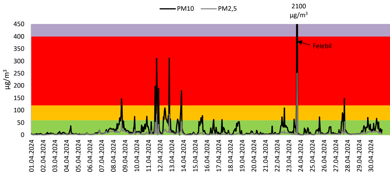
Figur 5-2. Timesmidler PM 10 og PM 2,5 ved Rektorhaugen i april 2024. Fargeklassifiseringen for varslingsklassene basert på helsevirkninger gjelder for PM 10 (svart linje). Grønn klasse: Liten eller ingen helserisiko, gul klasse: moderat helserisiko, rød klasse: betydelig helserisiko.
