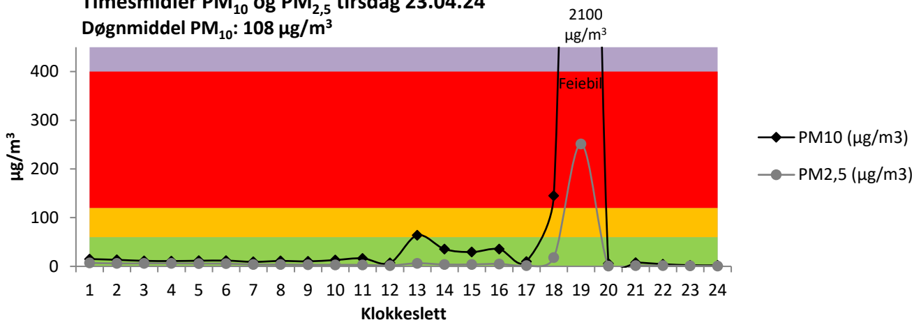
Figur 5-5 Timesmidler PM 10 og PM 2,5 for overskridelsesdøgn tirsdag 23.04.24. Fargeklassifiseringen for varslingsklassene basert på helsevirkninger gjelder for PM 10 (svart kurve).
