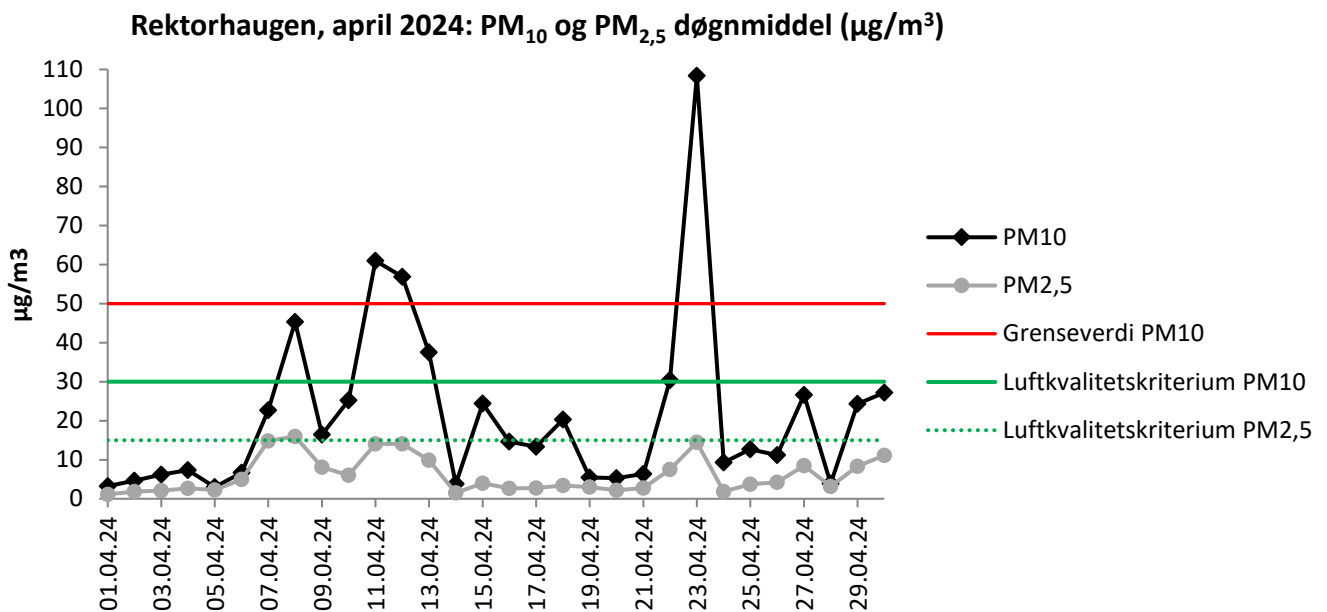
Figur 5-1. Døgnmidler PM 10 og PM 2,5 ved Rektorhaugen i april 2024, inkludert døgngrenseverdi for PM 10 på 50 µg/m 3 , og luftkvalitetskriteriene for døgnmidler PM 10 og PM 2,5 .
