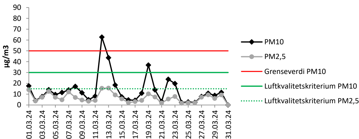
Figur 5-1. Døgnmidler \text{PM}_{10} og \text{PM}_{2,5} ved Rektorhaugen i mars 2024, inkludert døgngrenseverdi for \text{PM}_{10} på 50 \mu\text{g}/\text{m}^3 , og luftkvalitetskriteriene for døgnmidler \text{PM}_{10} og \text{PM}_{2,5} .
