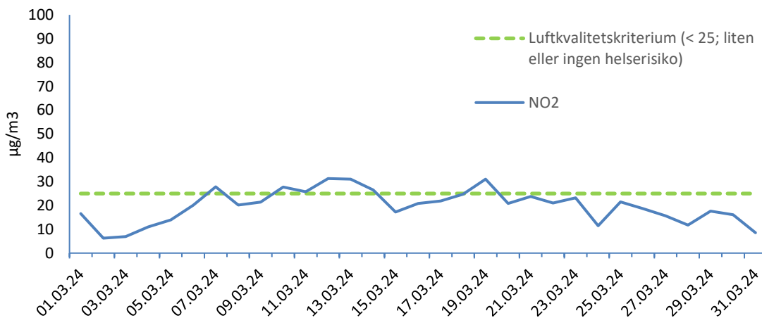
Figur 5-5. Målte døgnmidler NO 2 ved Rektorhaugen i mars 2024 sammen med luftkvalitetskriterium på 25 µg/m 3 .
