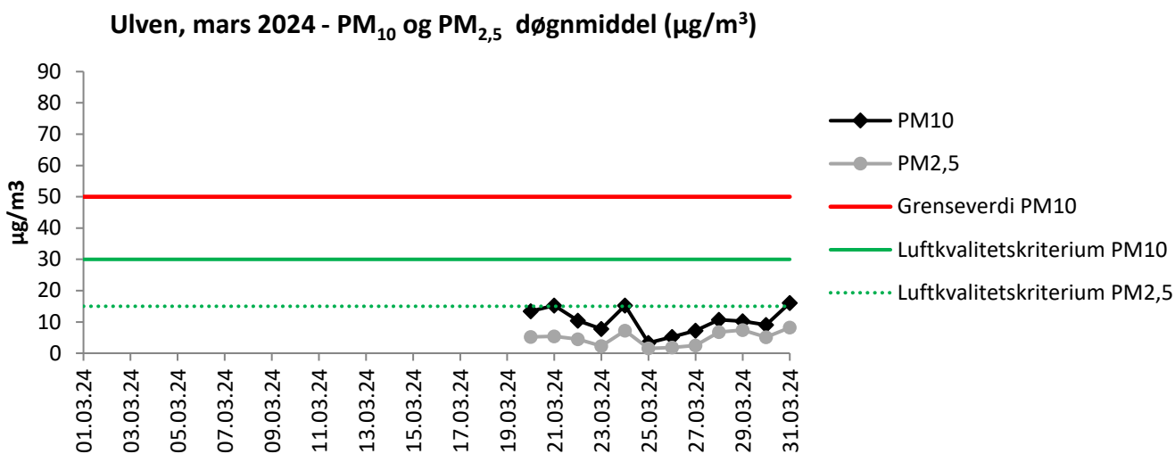
Figur 5-6 Døgngrænseverdier PM 10 og PM 2,5 ved Ulven i mars.
