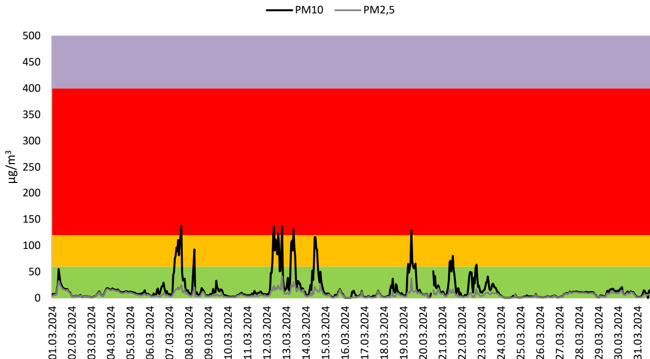
Figur 5-2. Timesmidler PM 10 og PM 2,5 ved Rektorhaugen i mars 2024. Fargeklassifiseringen for varslingsklassene basert på helsevirkninger gjelder for PM 10 (svart linje). Grønn klasse: Liten eller ingen helserisiko, gul klasse: moderat helserisiko, rød klasse: betydelig helserisiko.
