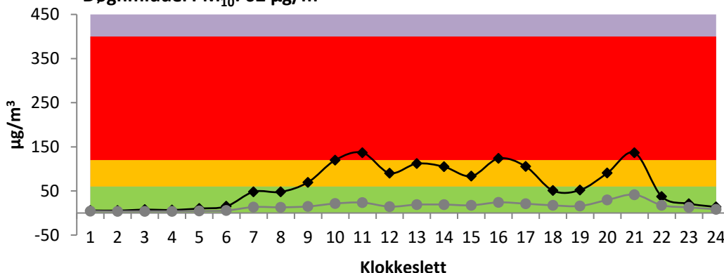
Figur 5-3 Timesmidler PM 10 og PM 2,5 for overskridelsesdøgn tirsdag 12.03.24. Fargeklassifiseringen for varslingsklassene basert på helsevirkninger gjelder for PM 10 (svart linje).
