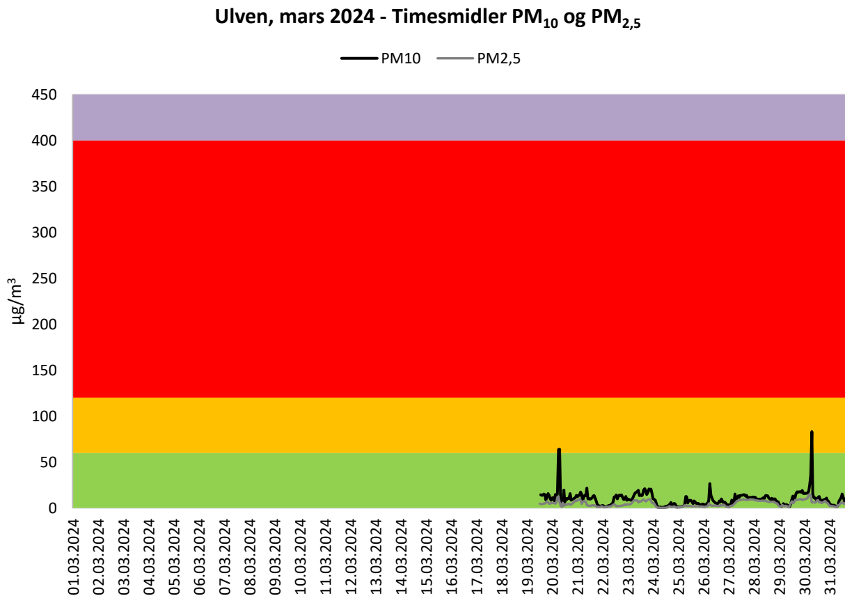
Figur 5-7 Timesmidler PM 10 og PM 2,5 ved Ulven i mars 2024. Fargeklassifiseringen for varslingsklassene basert på helsevirkninger gjelder for PM 10 (svart linje). Grønn klasse: Liten eller ingen helserisiko, gul klasse: moderat helserisiko, rød klasse: betydelig helserisiko.
