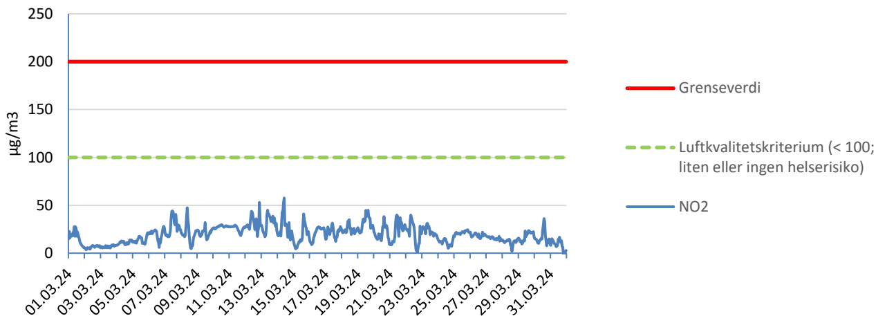
Figur 5-4. Målte timesmidler NO 2 ved Rektorhaugen i mars 2024 sammen med grenseverdi på 200 µg/m 3 og luftkvalitetskriterium på 100 µg/m 3 .
