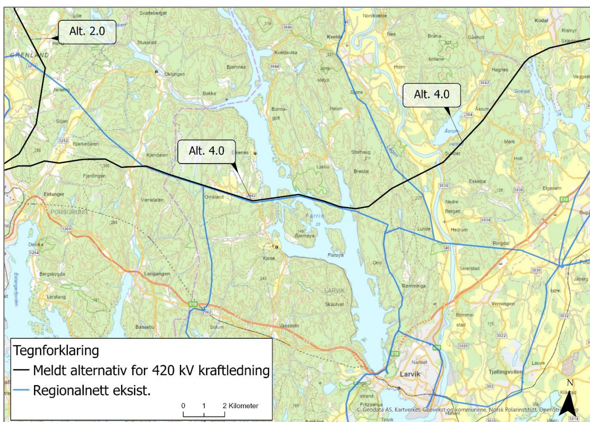
Figur 10 Oversikt alternativ 4.0. Alternativet følger på deler av strekningen eksisterende regionalnettledning.
