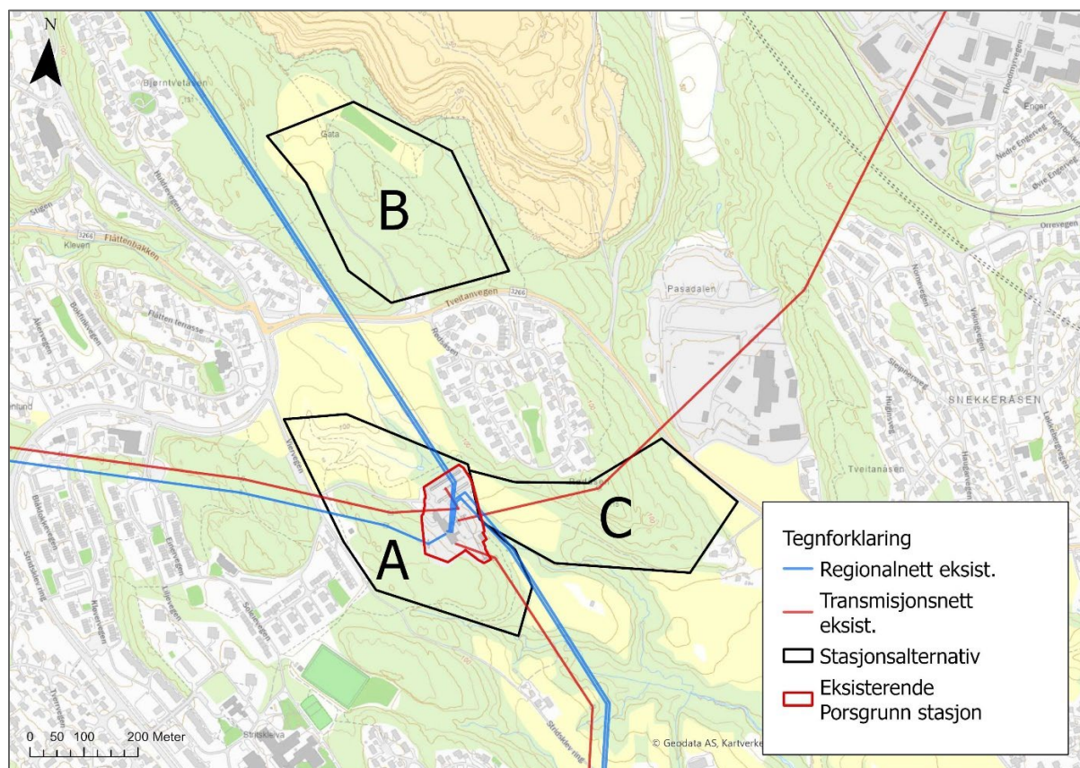
Figur 3 Alternative plasseringer av ny Porsgrunn transformatorstasjon. Areal i figur er betraktelig mye større enn ny stasjon, men hensyntar anleggsareal. Eksisterende transmisjons- og regionalnett (som vist i figur) må legges om som følge av ny transformatorstasjon.
