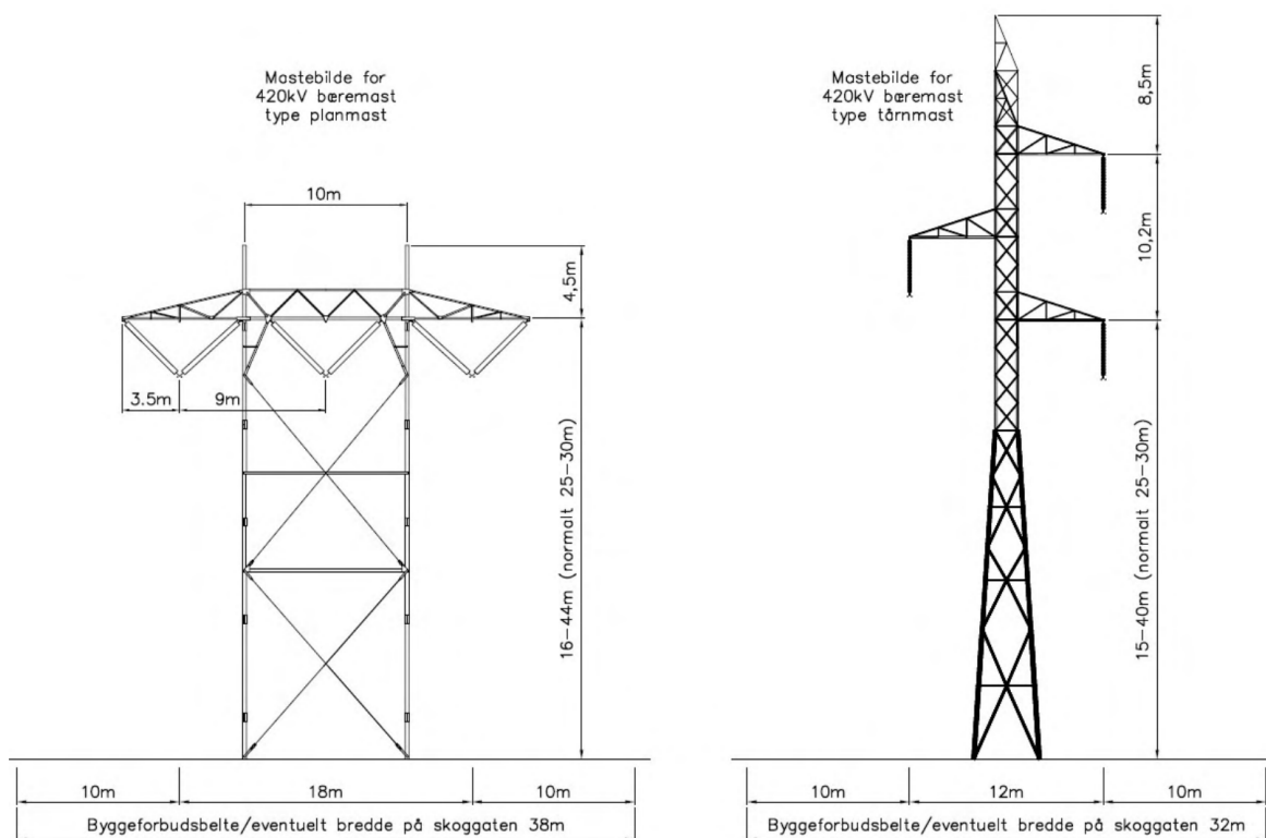
Figur 14 Illustrasjon av Statnetts standard bæremast til venstre og tårnmast til høyre.
