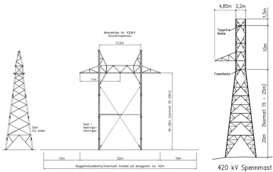
Figur 13 Illustrasjon av forankringsmast til venstre og fjordspennmast til høyre.
