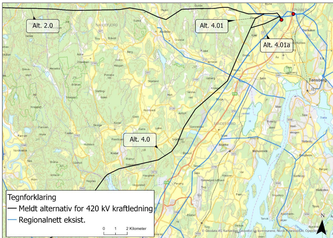
Figur 11 Oversikt alternativ 4.0, og alt. 4.01 og 4.01a inn mot Tønsberg transformatorstasjon (omsøkt 2023).
