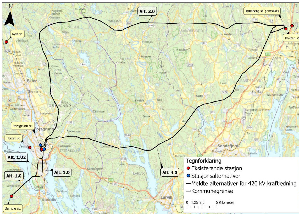
Figur 1 Alternativer for 420 kV forbindelse mellom Bamble, Porsgrunn og Tønsberg transformatorstasjon (omsøkt 2023). Meldte alternativ er markert med svart linje.
