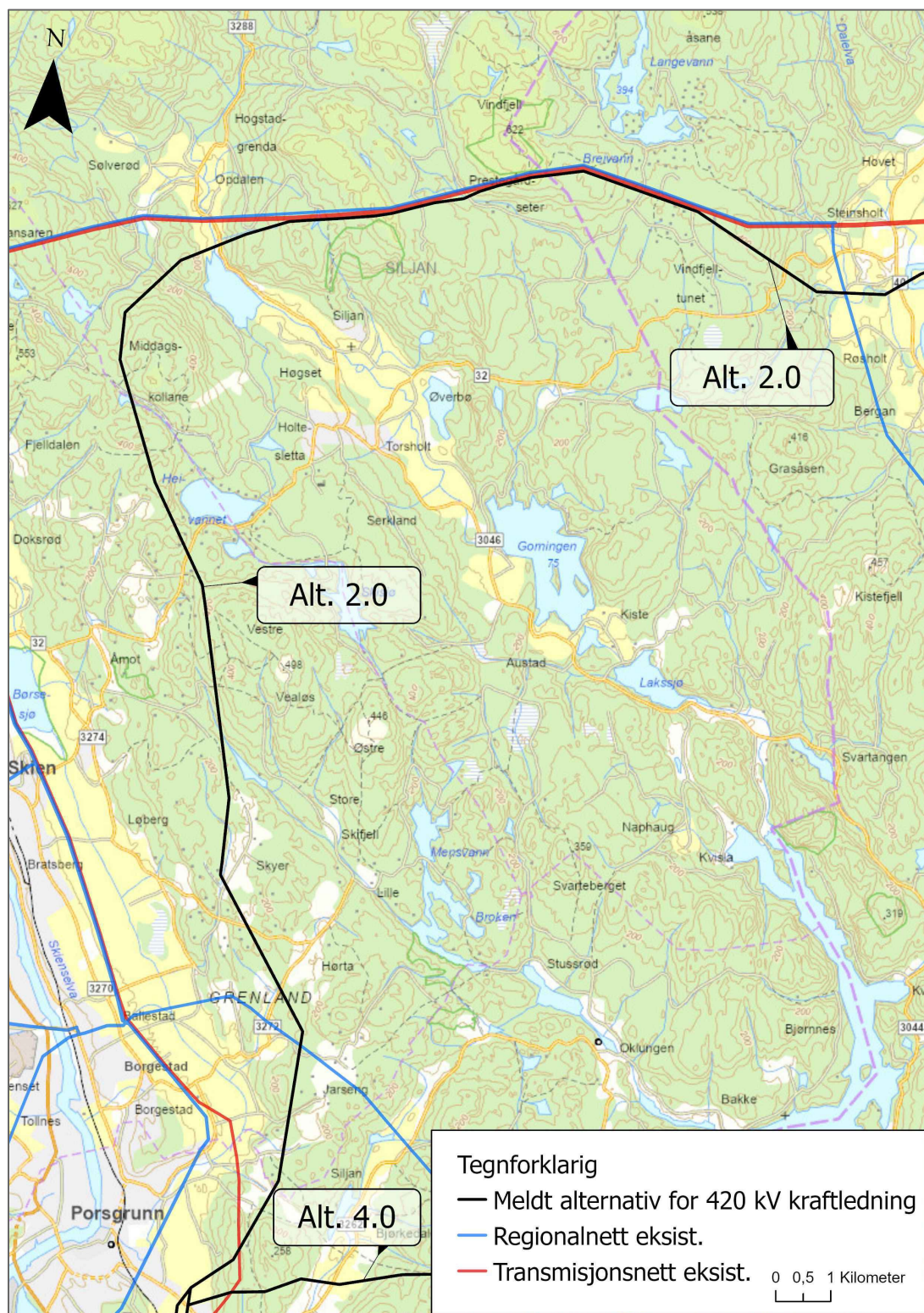
Figur 9 Oversikt alternativ 2.0 fra Porsgrunn til Steinsholt (Larvik kommune). Alternativet følger eksisterende regionalnett og transmisjonsnett på deler av strekningen fra nord for Opedalsvatnet i Siljan kommune.
