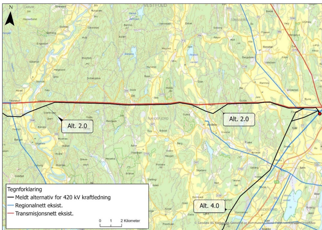
Figur 7 Oversikt alt. 2.0. Alternativet følger eksisterende transmisjonsnett (420 kV) på store deler av strekningen mellom Steinsholt og Tønsberg transformatorstasjon (omsøkt 2023).
