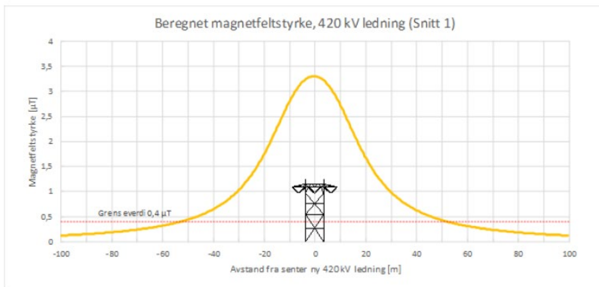
Figur 19 Eksempel på magnetfelt for en ny 420 kV kraftledning (ca. 370 MVA overføring).
