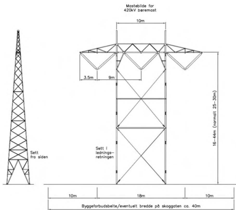
Figur 12 Illustrasjon av Statnetts standard 420 kV bæremaster.
