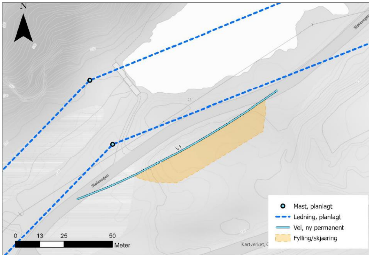
Figur 3-1. Det er planlagt en justering av Stølevegen for å få plass til et av mastepunktene.
