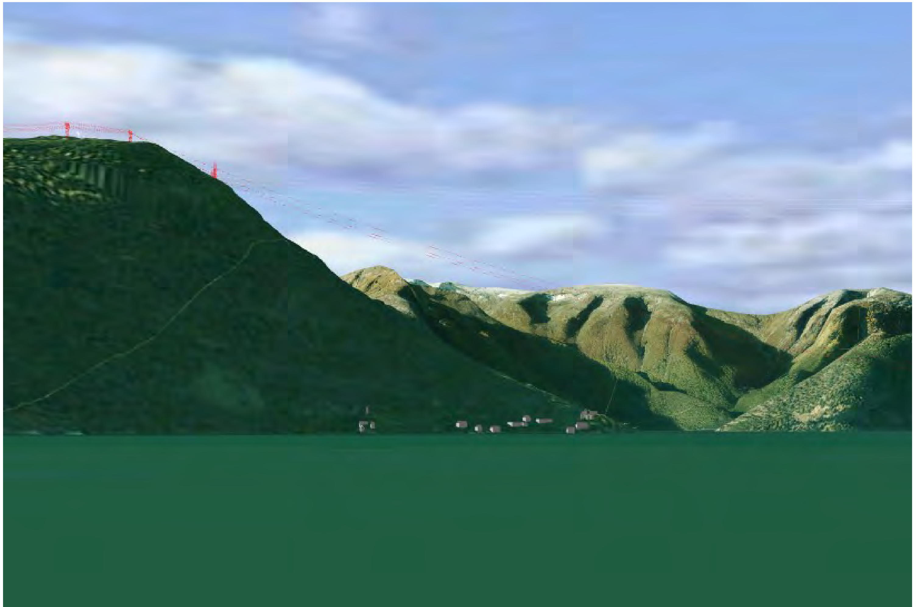
Modellbilde av Frønningen, eksisterende ledning, som skal rives, i rødt, og ny ledning i hvitt.
