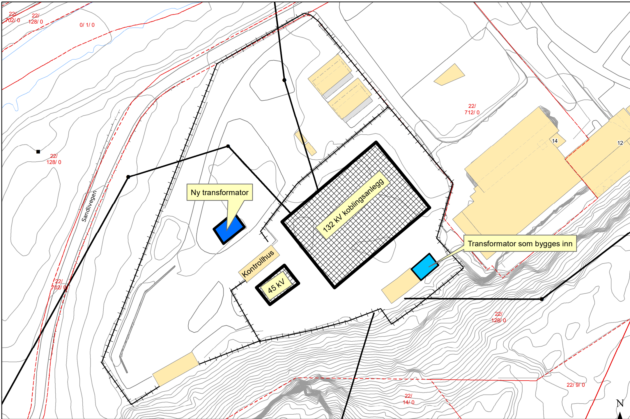
Dale transformatorstasjon - situasjonsplan
