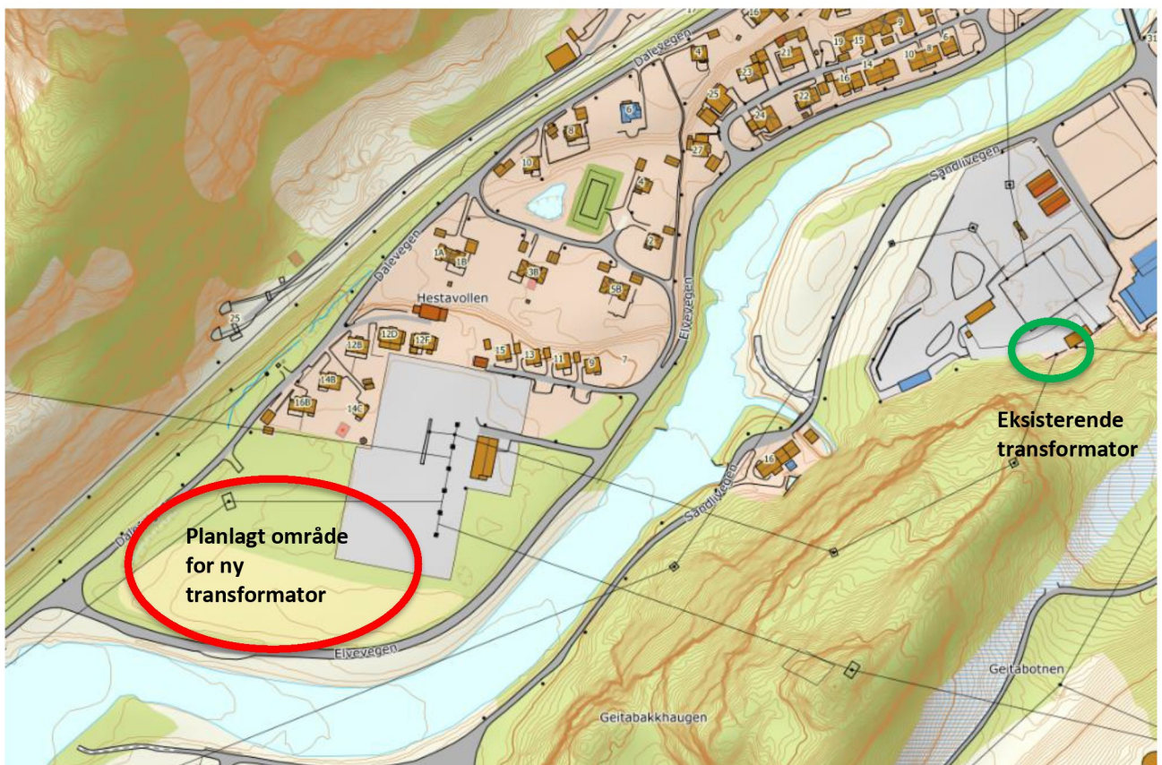
Figur 1 Markering av planlagt nytt område for transformator er markert med rød heltrukket linje, og markering av plassering av eksisterende transformator er markert med grønn heltrukket linje [norgeskart.no].
