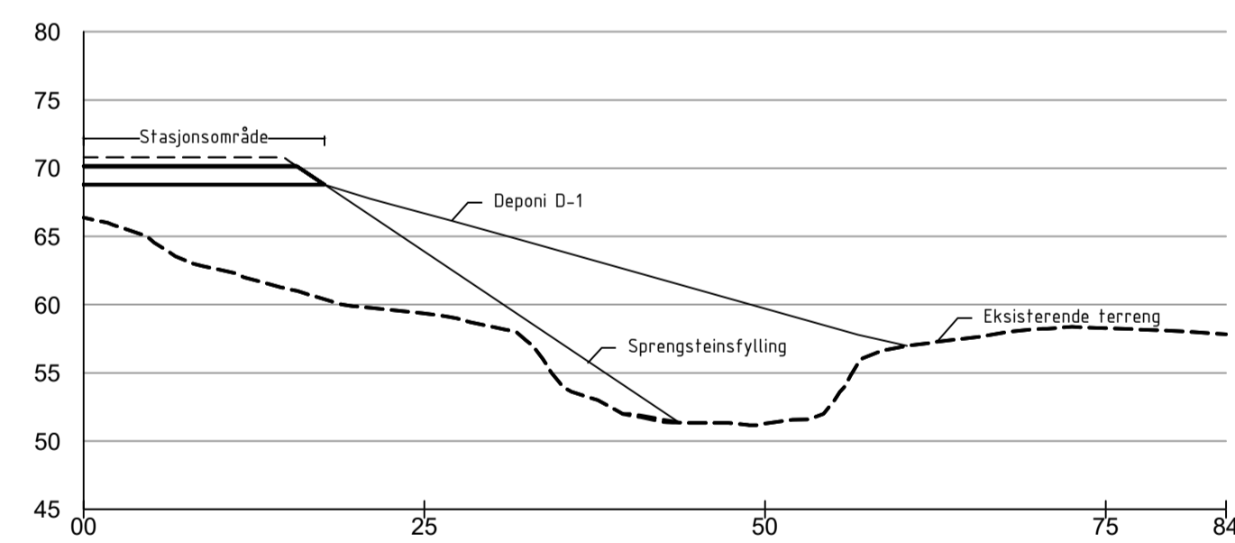
Deponi D-1 - Snitt B
