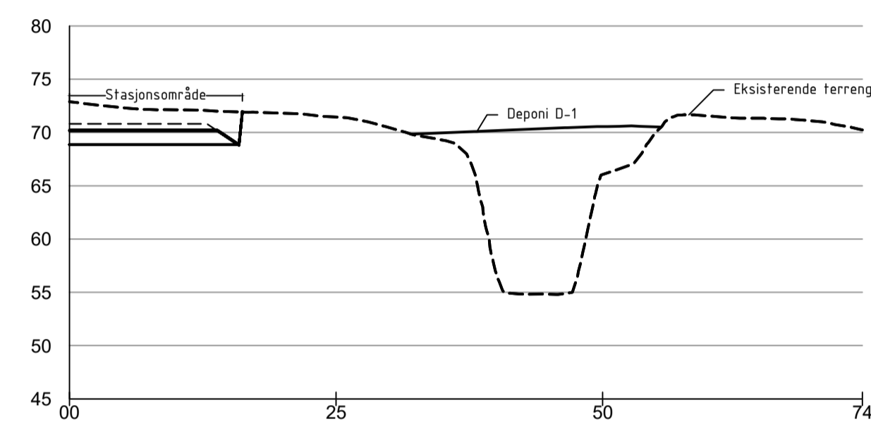
Deponi D-1 - Snitt A
