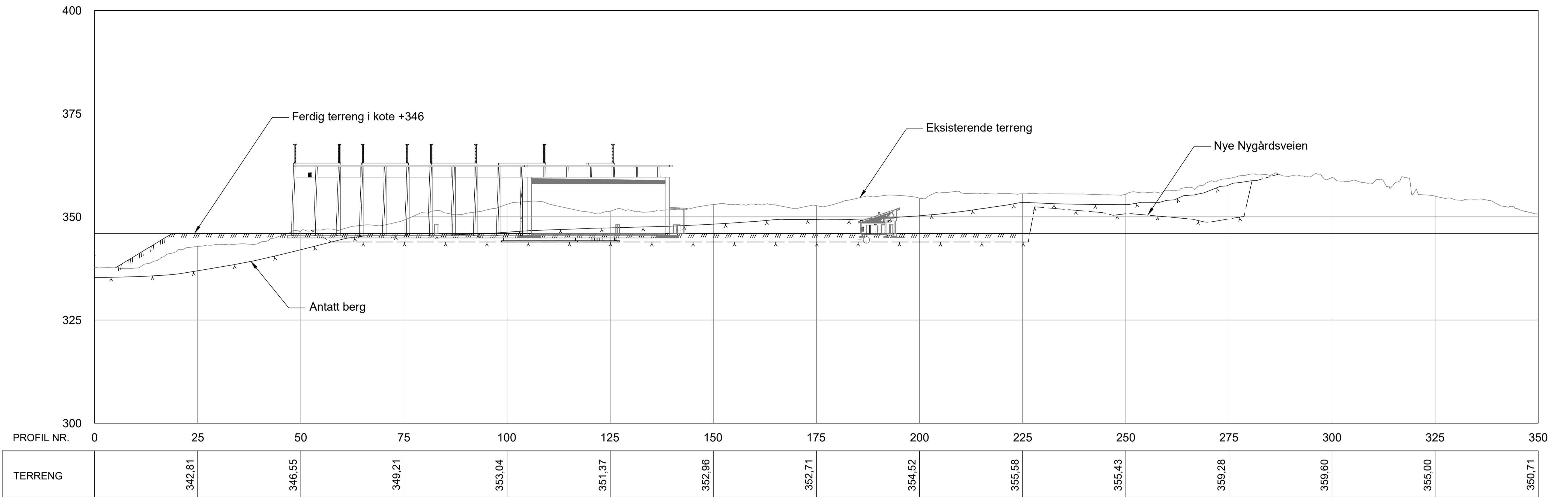
Lengdesnitt 1:500
