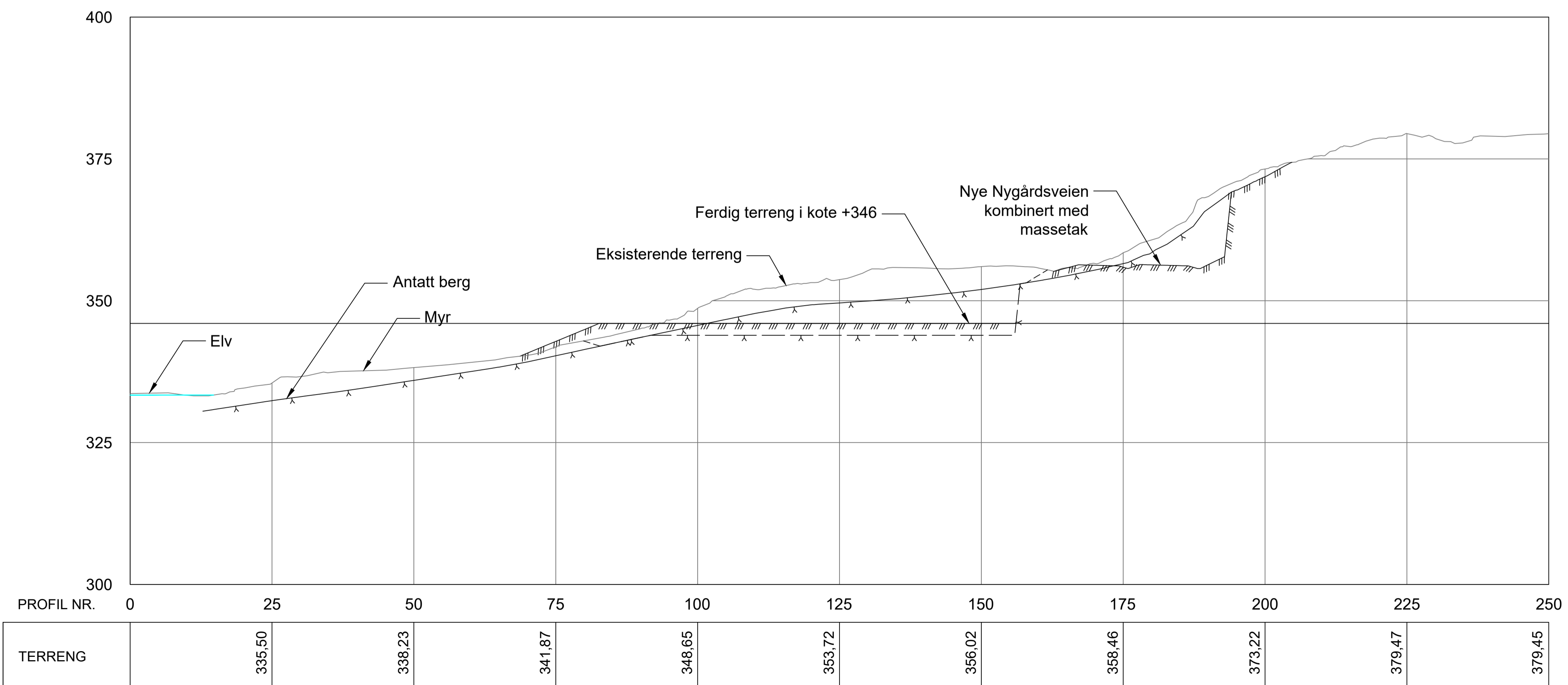
Tversrsnitt 1:500
